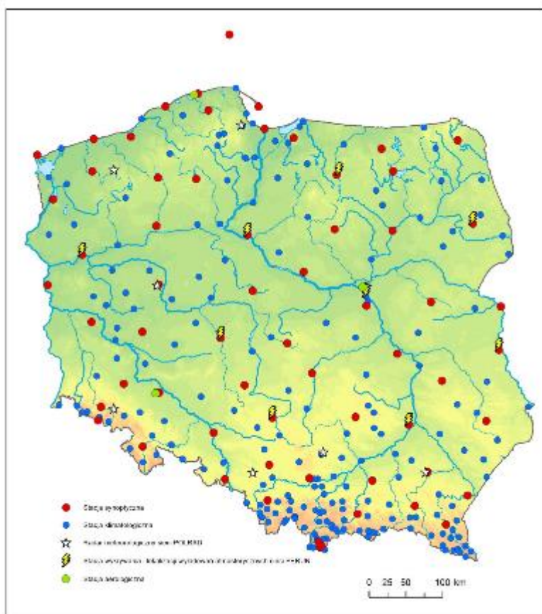
Rys. 8.1. Sieć obserwacyjnyjny IMGW-PIB (stan na 1.01.2022 r.)
