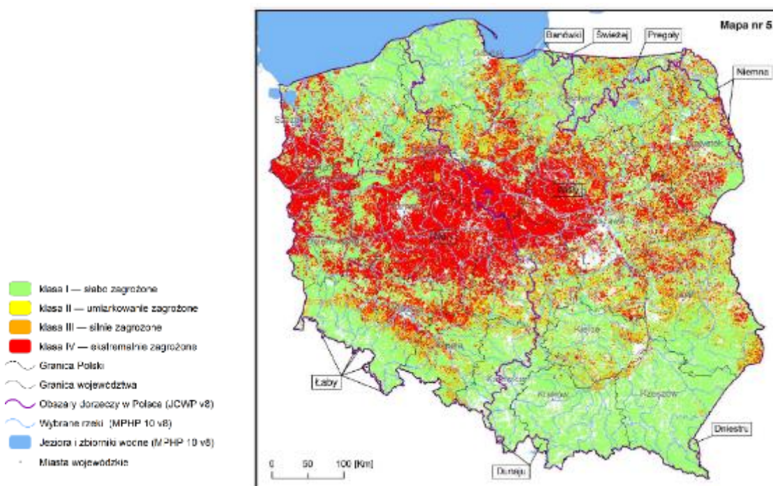
Rys. 6.27. Zagrożenie suszą rolniczą na terenach rolnych i leśnych
