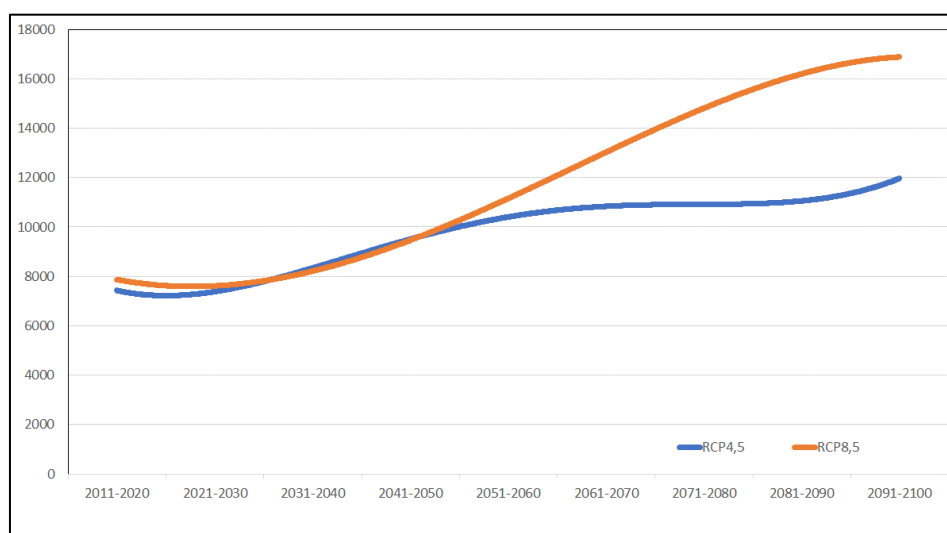
Rys. 6.15. Liczba osób w Polsce z wysokim i bardzo wysokim ryzykiem zagrożenia upałami
