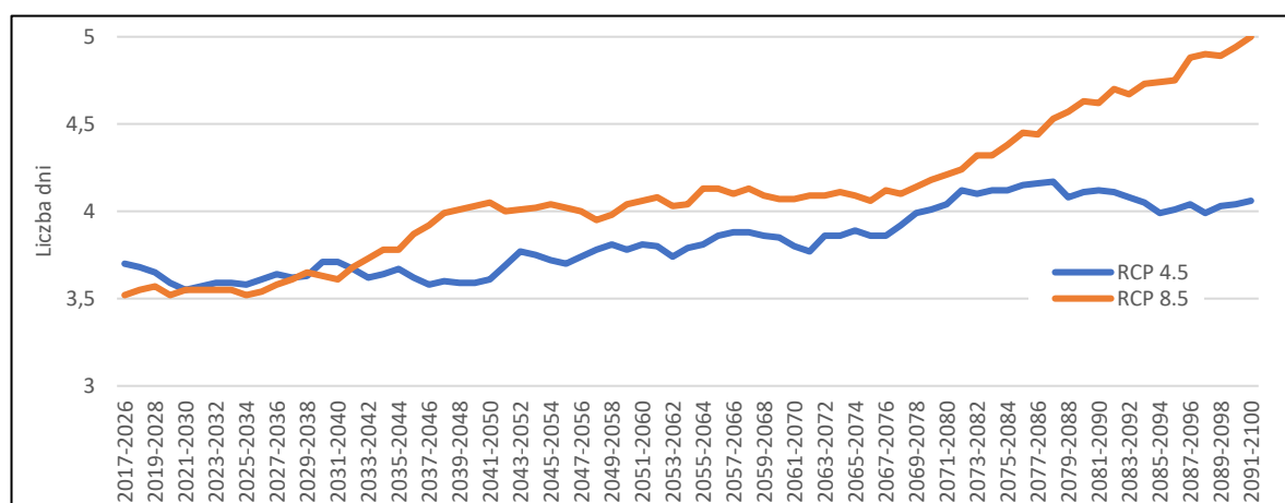
Rys. 6.11. Roczna liczba dni z opadem >20 mm w Polsce w okresie 2017-2100 dla scenariuszy RCP8.5 i RCP 4.5
