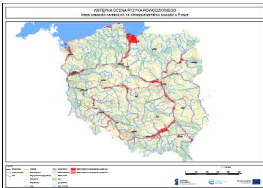
Rys. 6.25. Obszary narażone na niebezpieczeństwo powodzi w Polsce
