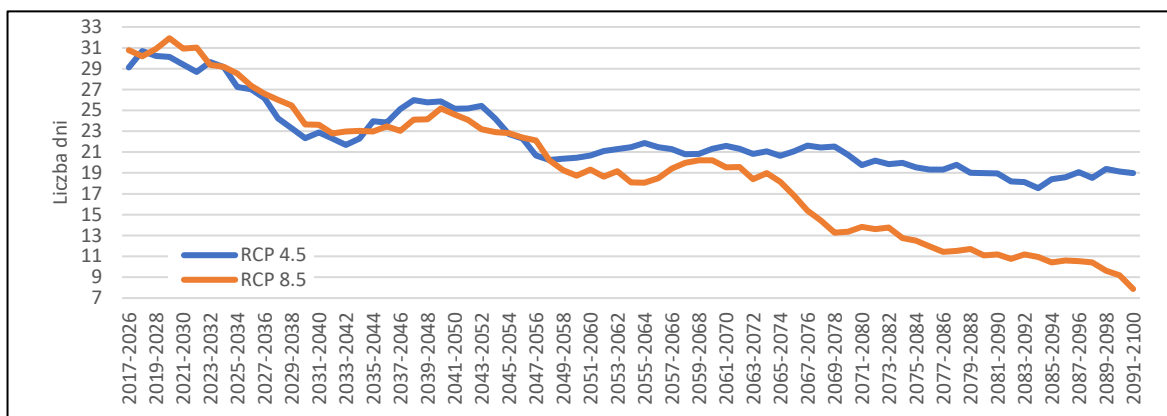
Rys. 6.7. Roczna liczba dni z temperaturą maksymalną <0^{\circ}\text{C} w Polsce w okresie 2017-2100 dla scenariuszy RCP 8.5 i RCP 4.5
