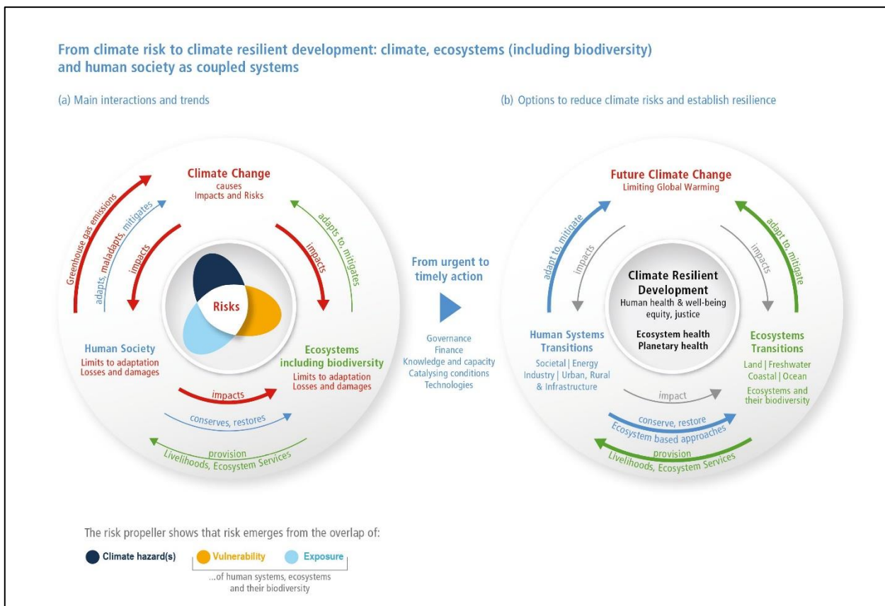
Rys. 6.13. Ogólny schemat integracji i powiązań zmian ryzyka związanego ze zmianami klimatu ze wskazaniem elementów zagrożenia, ekspozycji oraz podatności w klimacie obecnym i przyszłym
