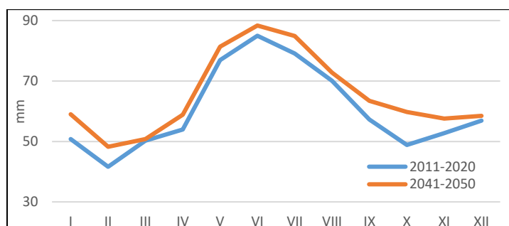
Rys. 6.9. Miesięczna suma opadu w Polsce w latach 2011-2020 i 2041-2050 w scenariuszu RCP 8.5
