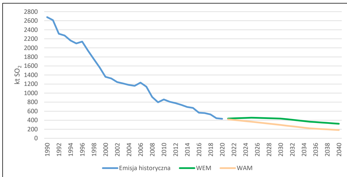
Rys. 5.9. Emisja historyczna SO 2 w latach 1990-2020 oraz prognozowane wielkości emisji do 2040 r. wg scenariuszy WEM i WAM
