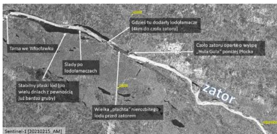
Rys. 8.7. Przykład analizy obrazu Sentinel-1/SAR) polaryzacja VV) pod kątem detekcji zatorów lodowych na rzece. Zator lodowy na Wiśle w okolicach Płocka, 15.02.2021 r.
