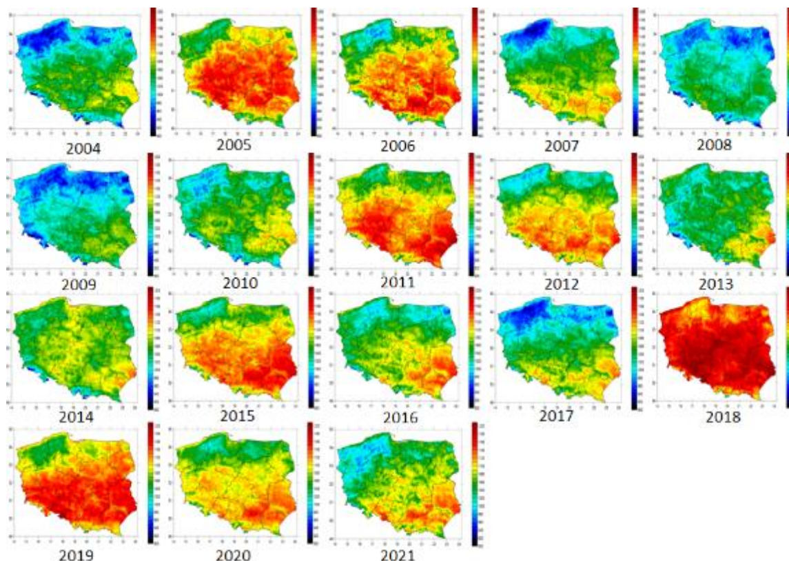
Rys. 8.13. Rozkład przestrzenny nasłonecznienia w latach 2004-2021 (sumy roczne w kWh/m²)
