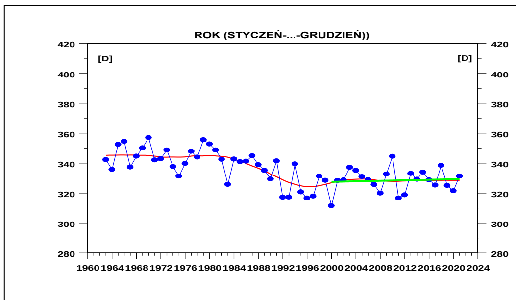
Rys. 8.14. Średnie całkowitej zawartości ozonu uzyskane z pomiarów spektrofotometrem Dobsona w COG IGF PAN, Belsk, w okresie 1963-2021. Krzywa czerwona przedstawia wygładzone dane, a zielona liniowy trend (nieistotny statystycznie) w okresie 2000-2021.
