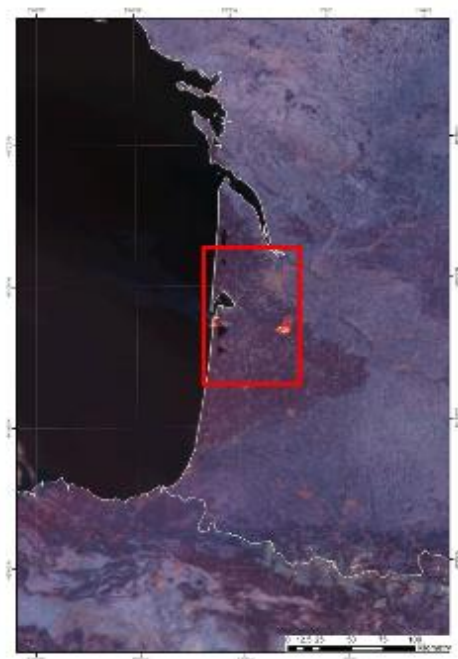
Rys. 8.10. Kompozycja RGB Fire temperature (R=3.9μm; G=2.2μm; B=1.6μm), S-NPP/VIIRS z dnia 18.07.2022 r., 11:43 UTC. Widoczny pożar lasów (jasno pomarańczowy i żółty kolor) na pld. od Bordeaux we Francji.
