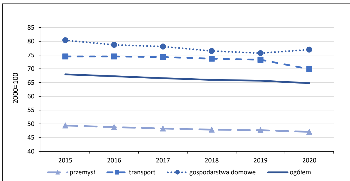
Rys. 2.13. Wskaźnik ODEX 2015-2020 (2000=100)
