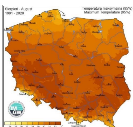
Rys. 6.29. Wartości maksymalnej dobowej temperatury powietrza o prawdopodobieństwie wystąpienia 5% w wybranych miesiącach
