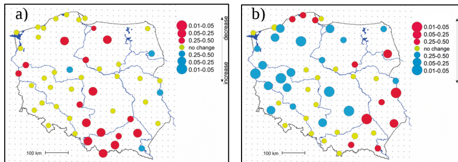
Rys. 6.3. Poziom istotności zmian udziału opadów letnich (JJA) do rocznych w okresach 1951-2013 (a) i opadów zimowych (DJF) do opadów rocznych w okresach 1952-2013 na podstawie testu Manna-Kendalla
