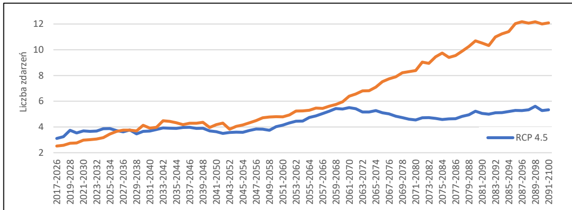
Rys. 6.6. Roczna liczba dni z temperaturą minimalną >20^{\circ}\text{C} w Polsce w okresie 2017-2100 dla scenariuszy RCP 8.5 i RCP 4.5
