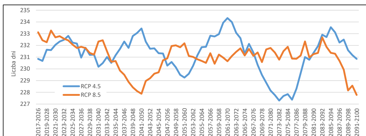
Rys. 6.10. Roczna liczba dni bez opadu w Polsce w okresie 2017-2100 dla scenariuszy RCP 8.5 i 4.5
