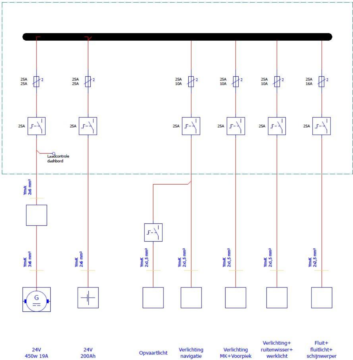
Przykład 2 Tablica rozdzielcza w sterówce 24 V
