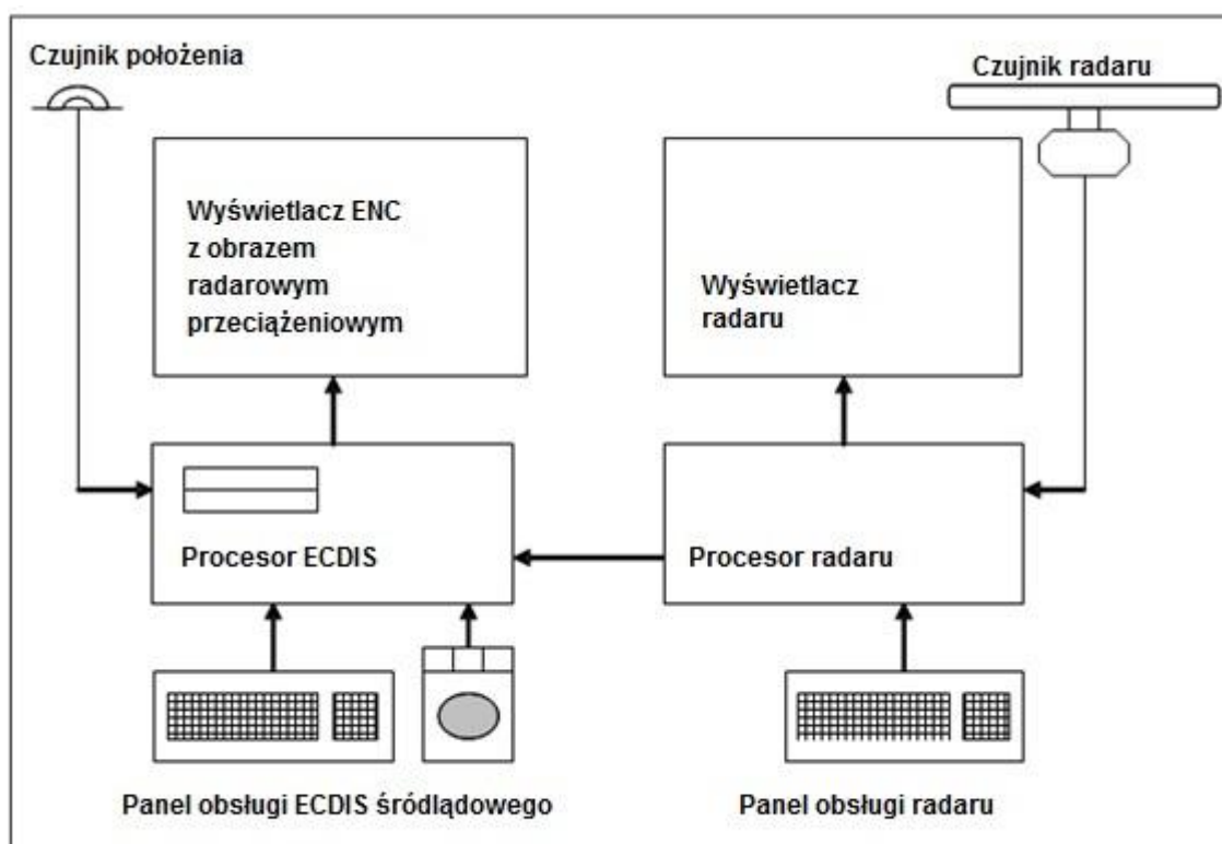
Rysunek 1 Sprzęt ECDIS śródlądowego, niezależny sprzęt podłączony do sprzętu radarowego (konfiguracja systemu 2)
