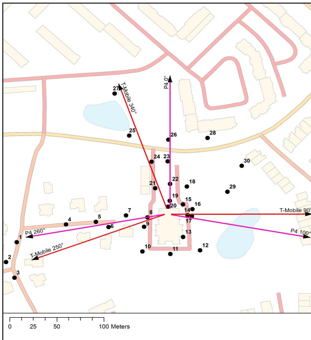
Rys. 1: Plan terenu, na którym znajdują się badane stacje bazowe
