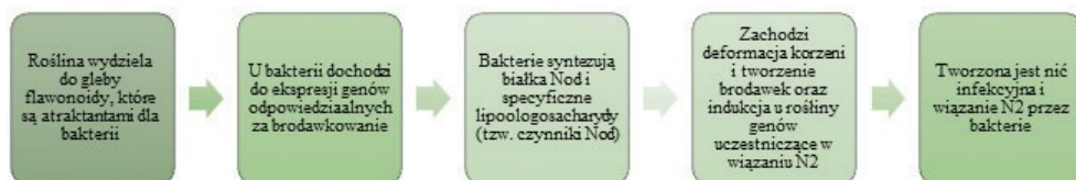
Rys 1. Etapy biologicznego wiązania azotu (na podstawie: Łyszcz i Gałązka 2016)
