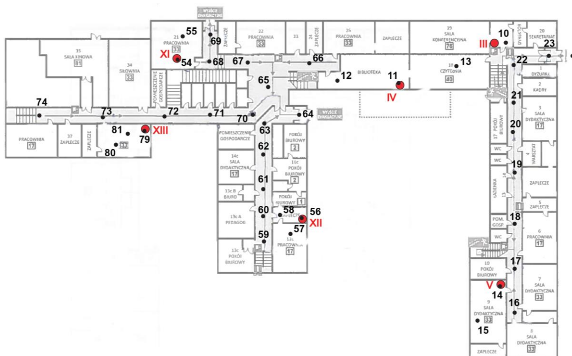
Rys. 1b: Plan rozmieszczenia punktów pomiarowych – parter kolorem czerwonym oznaczono lokalizację punktów dostępowych
