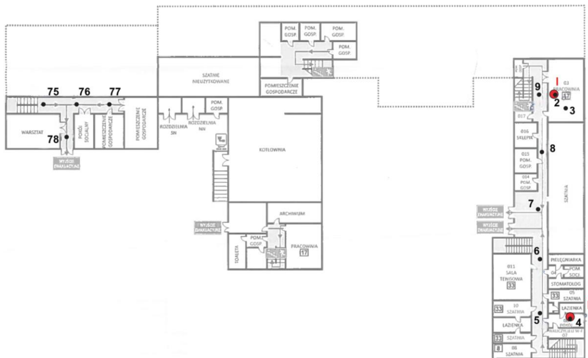
Rys. 1a: Plan rozmieszczenia punktów pomiarowych – piwnica kolorem czerwonym oznaczono lokalizację punktów dostępowych
