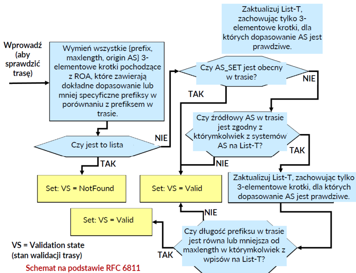
Rysunek 7: Algorytm sprawdzania pochodzenia (na podstawie RFC 6811)
