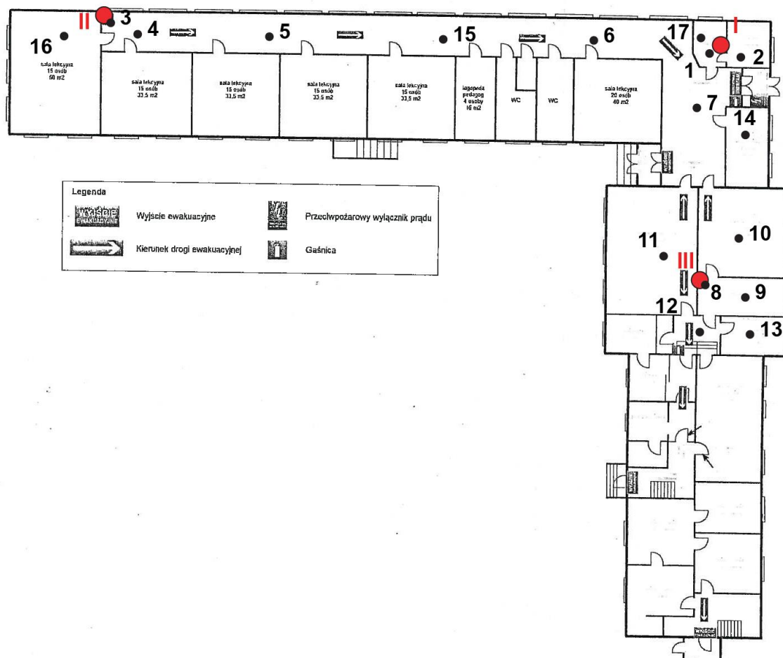
Rys. 1: Plan rozmieszczenia punktów pomiarowych
