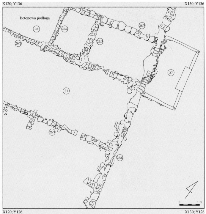
8. Zarys fundamentów dworu w Mielewszczyźnie – faza III użytkowania majądanu. Rys. G. Nowakowska. Outline of the foundations of a manor house in Mielewszczyzna – phase III of using the courtyard. Drawing: G. Nowakowska.
