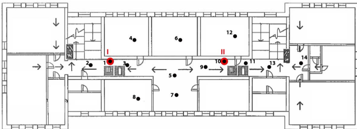
Rys. 1d: Plan rozmieszczenia punktów pomiarowych – II piętro, kolorem czerwonym oznaczono lokalizację punktów dostępowych
