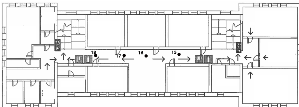
Rys. 1c: Plan rozmieszczenia punktów pomiarowych – I piętro
