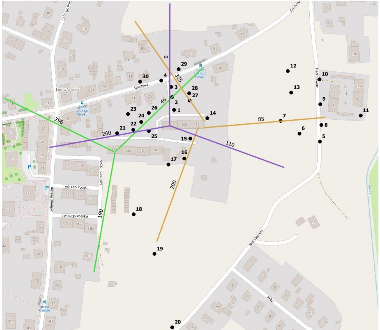
Rys. 1: Plan terenu, na którym znajdują się badane stacje bazowe
