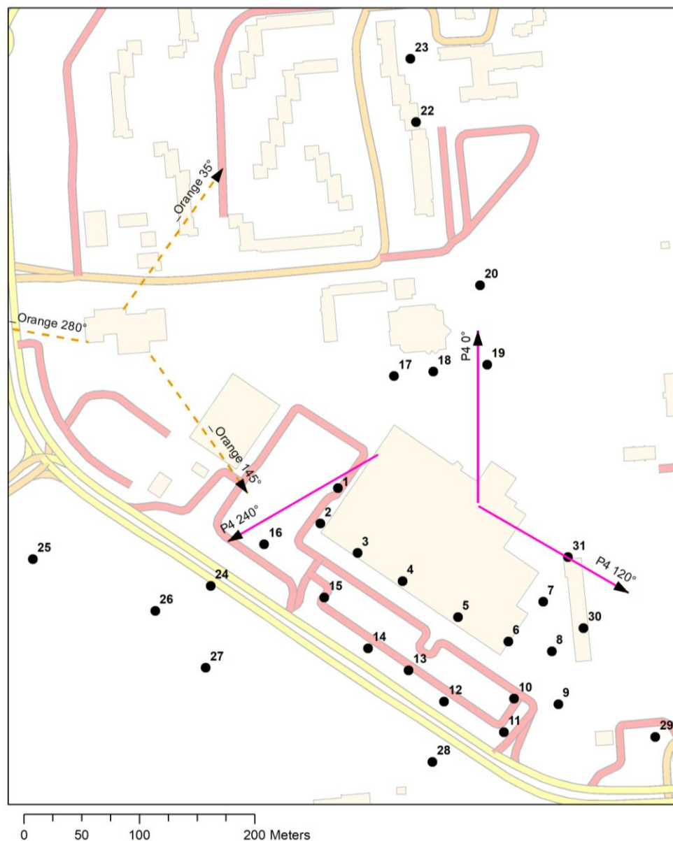
Rys. 1: Plan terenu, na którym znajdują się badana stacja bazowa
