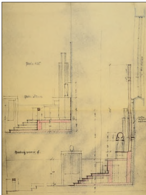
9. Karta z projektu ołtarza głównego autorstwa I. Kędzierskiego, 1946 r., przekrój boczny, w archiwum parafii pw. św. Michała Archaniola w Lublinie
