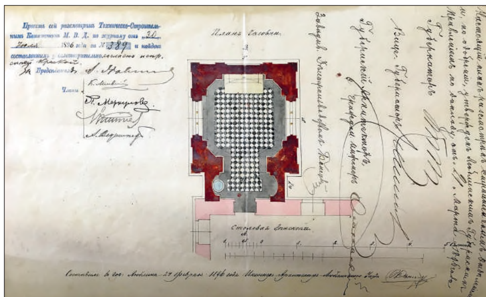
6. Projekt kaplicy domowej biskupa F. Jaczewskiego z 1896 r., rzut. Archiwum Państwowe w Lublinie, Rząd Gubernialny Lubelski, Referat IV Wyznaniowy, sygn.: 14240.
