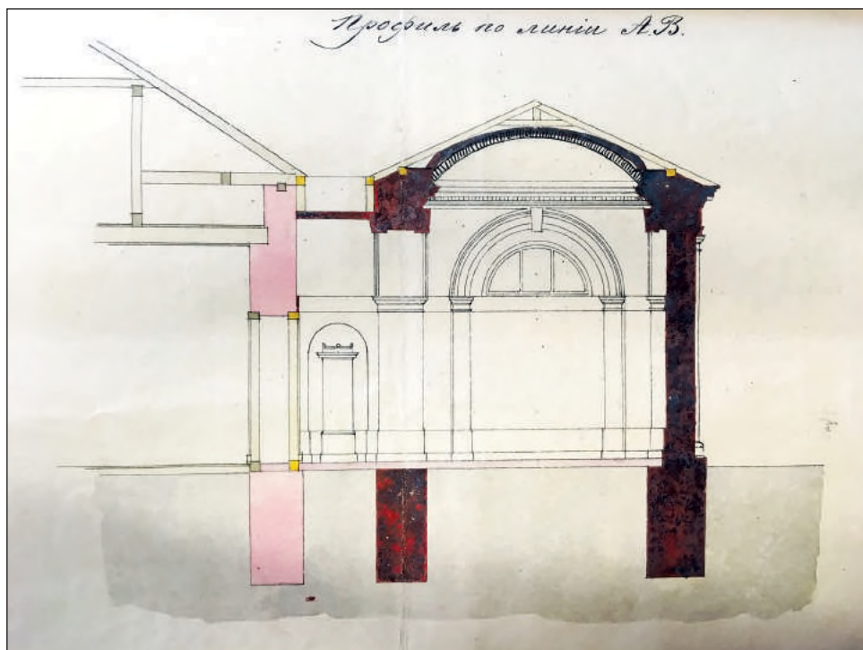
5. Projekt kaplicy domowej biskupa F. Jaczewskiego z 1896 r., przekrój. Archiwum Państwowe w Lublinie, Rząd Gubernialny Lubelski, Referat IV Wyznaniowy, sygn.: 14240.
