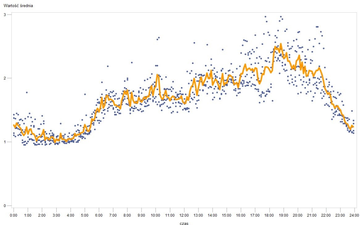
Rys. 7 Wyniki pomiarów – SP nr 22 we Wrocławiu – średnia za okres 24 godzin
