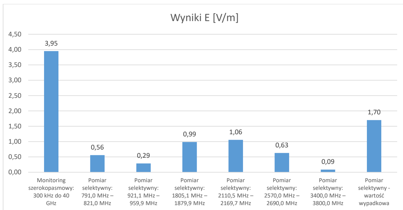
Rys. 15 Porównanie wyników monitoringu szerokopasmowego i pomiarów selektywnych
