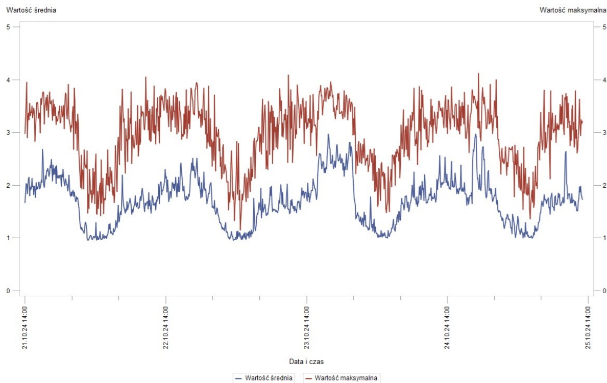
Rys. 6 Wyniki pomiarów – SP nr 22 we Wrocławiu w dniach 21.10.2024 r. – 25.10.2024 r. – wartość średnia i wartość maksymalna
