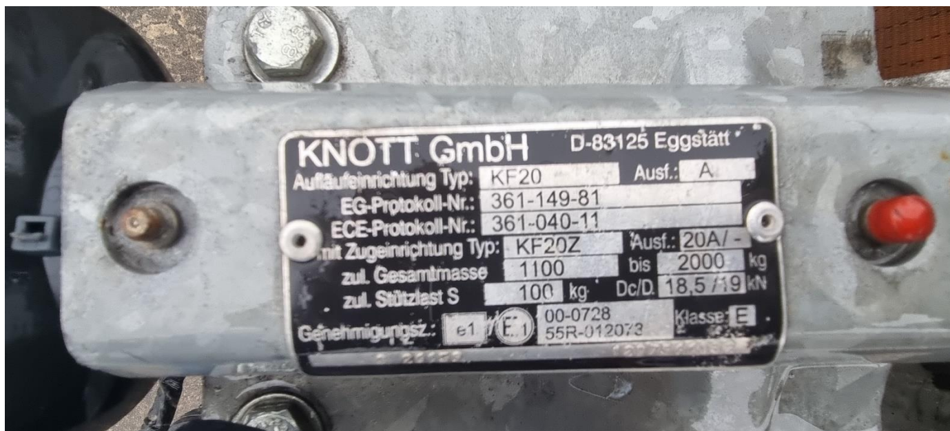
Foto nr 27 Łódź ŁM OIRM 1 –przyczepa podłodziowa tabliczka znamionowaw dniu 06.05.2026
