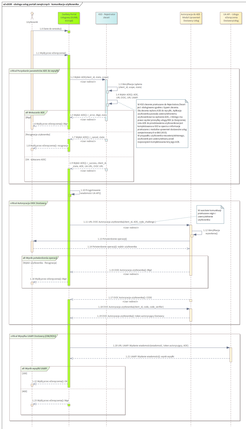
Rysunek 2 Diagram sekwencji dla wysyłki z systemu usługowego z użyciem usługi RDE
