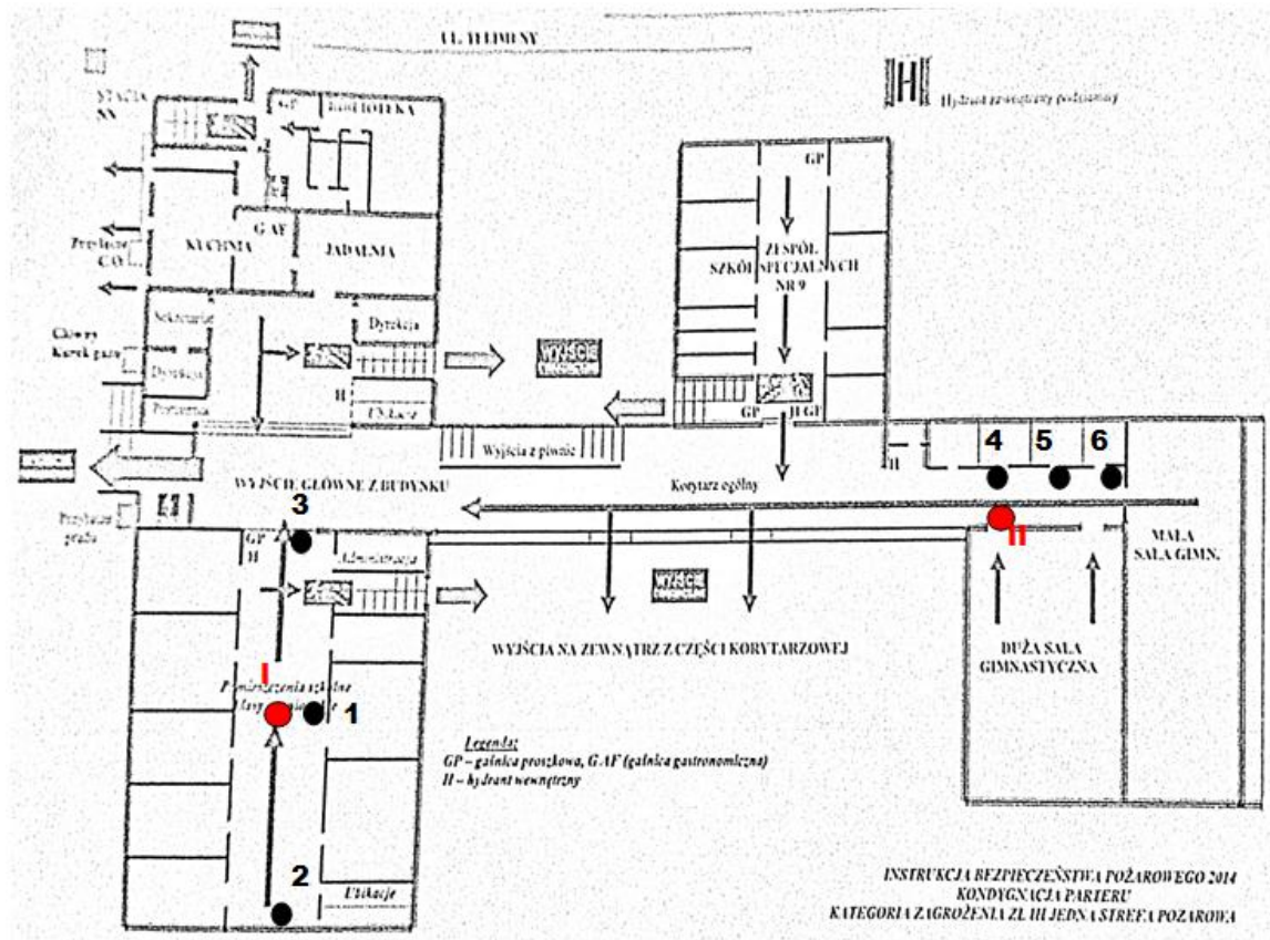
Rys. 1a: Plan rozmieszczenia punktów pomiarowych – parter, kolorem czerwonym oznaczono lokalizację punktów dostępnych
