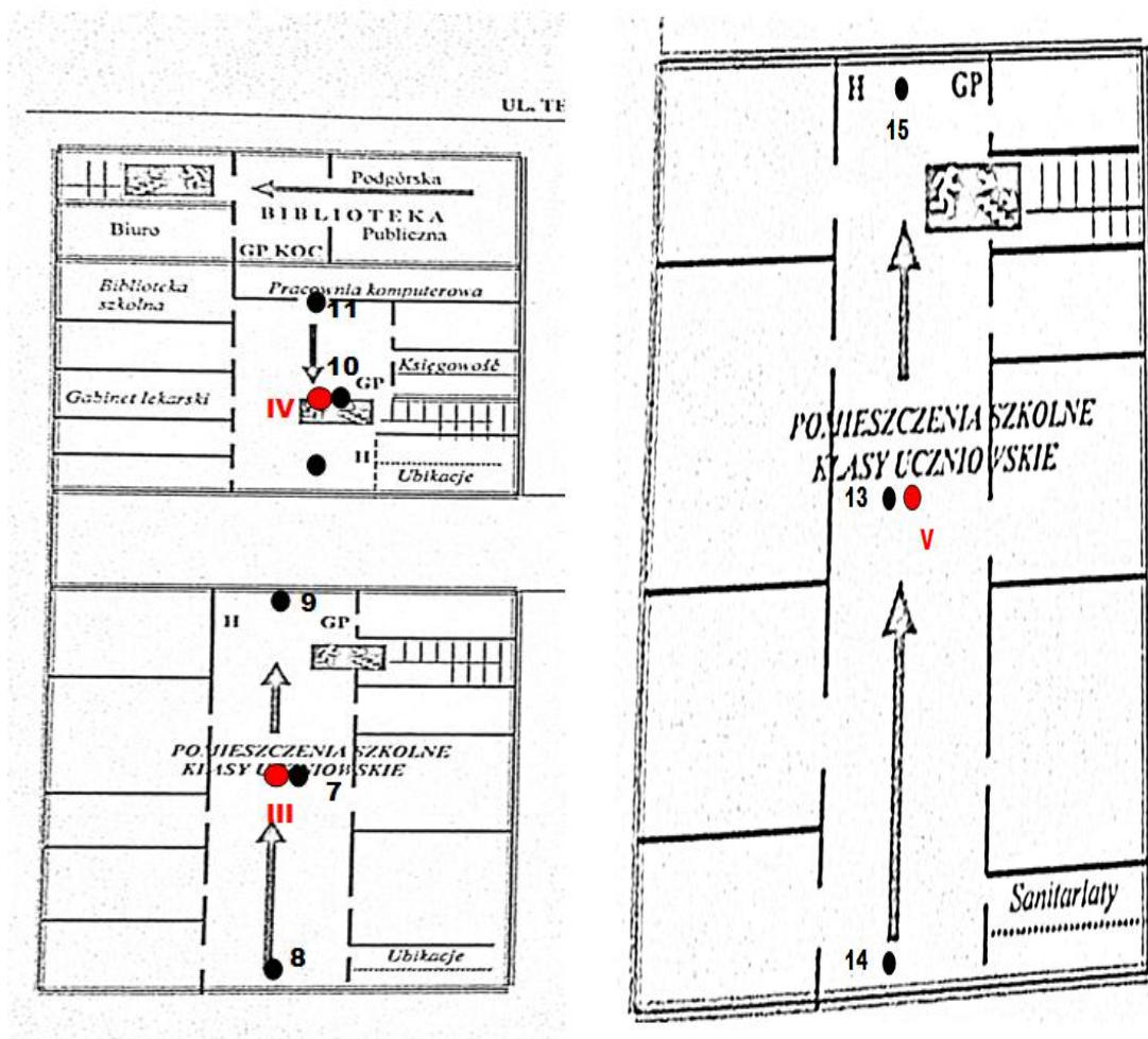
Rys. 1b, c: Plan rozmieszczenia punktów pomiarowych – 1 piętro (po lewej) oraz 2 piętro (po prawej), kolorem czerwonym oznaczono lokalizację punktów dostępowych
