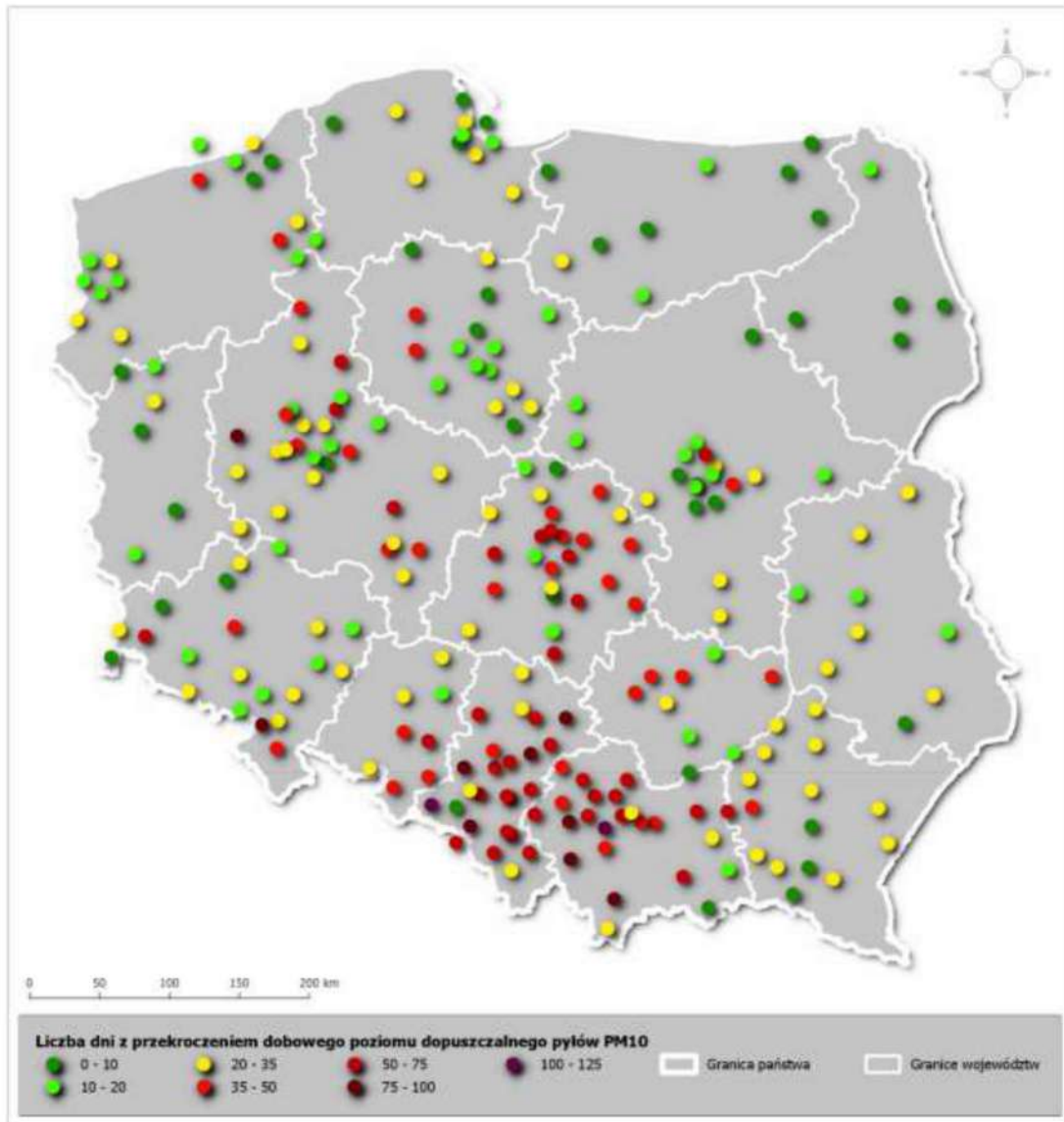
Rysunek 6. Liczba dni z przekroczeniem poziomu dopuszczalnego dobowego stężenia pyłu PM10 w 2019 roku na stanowiskach pomiarowych PMŚ 41
