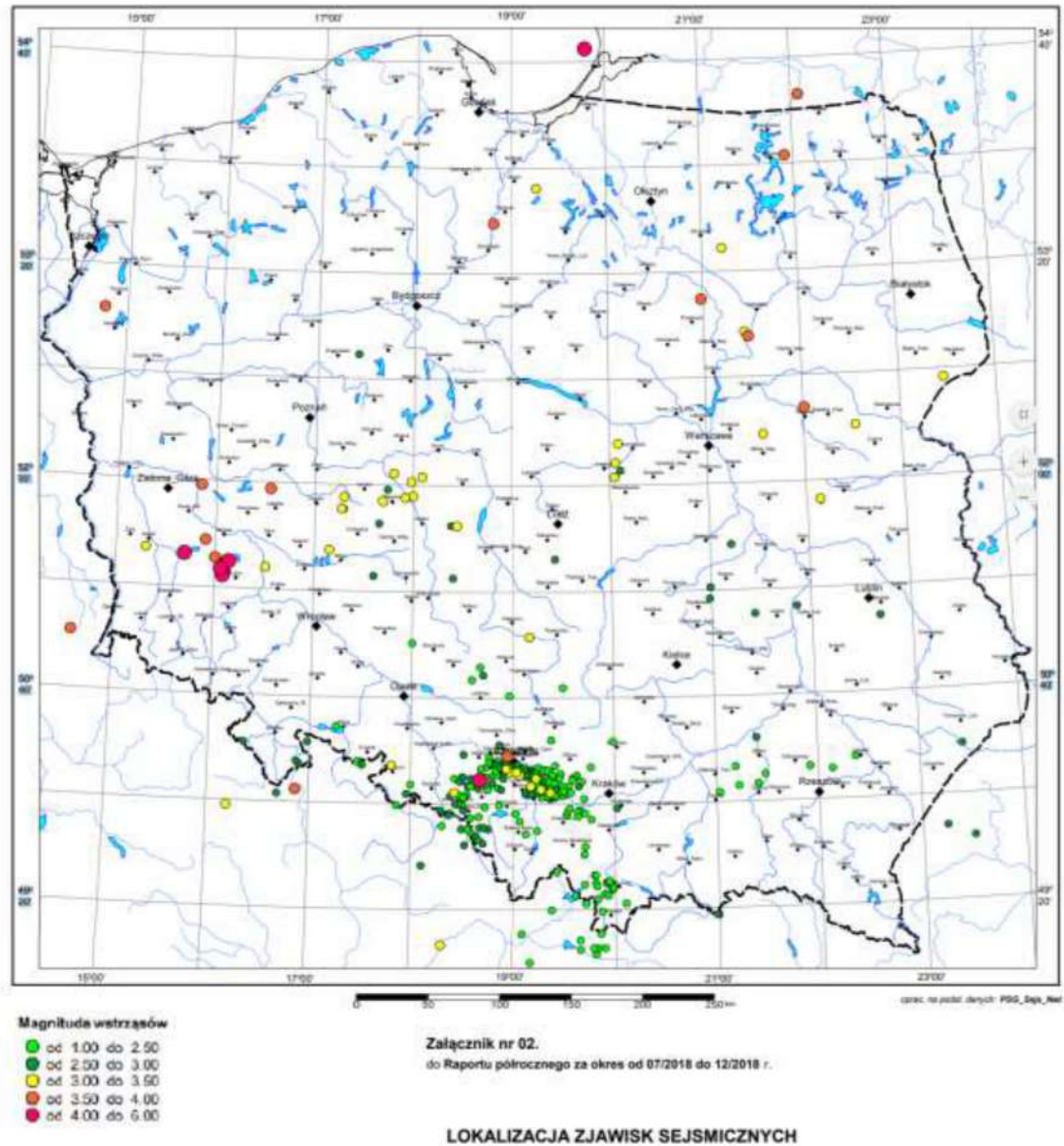
Rysunek 76. Lokalizacja zjawisk sejsmicznych na obszarze Polski wykrytych przez system automatycznego alertowania sieci monitoringu sejsmicznego PSG_Sejs_Net w okresie od 01/07/2018 do 31/12/2018 r. 170
