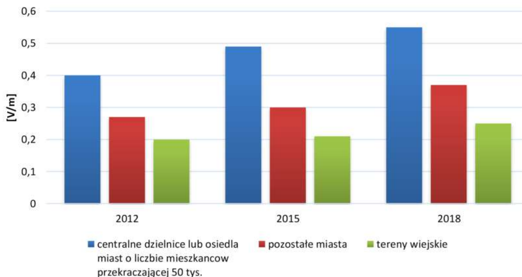
Rysunek 42. Zmiana średniego natężenia składowej elektrycznej uzyskanej na poszczególnych obszarach w tych samych lokalizacjach w kolejnych cyklach pomiarowych (lata 2012, 2015 i 2018) 109
