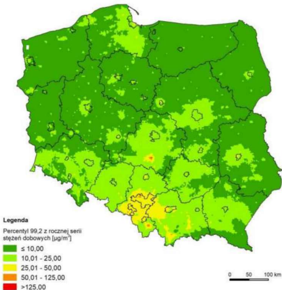
Rysunek 14. Rozkład przestrzenny stężeń \text{SO}_2 wyrażony jako percentyl 99,2 z rocznej serii stężeń dobowych na obszarze Polski w 2018 roku określony na podstawie modelowania matematycznego 51
