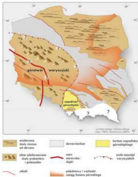
Rysunek 57. Rozmieszczenie formacji skalnych na terenie Polski bez osadów permu, mezozoiku i kenozoiku 140
