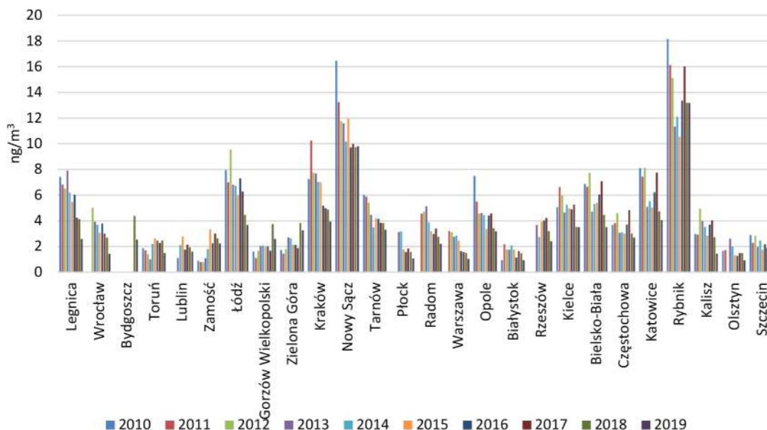
Rysunek 12. Trend zmian w wysokości stężeń benzo(a)pirenu na stacjach pomiarowych w wybranych miastach kraju w latach 2010-2019 49
