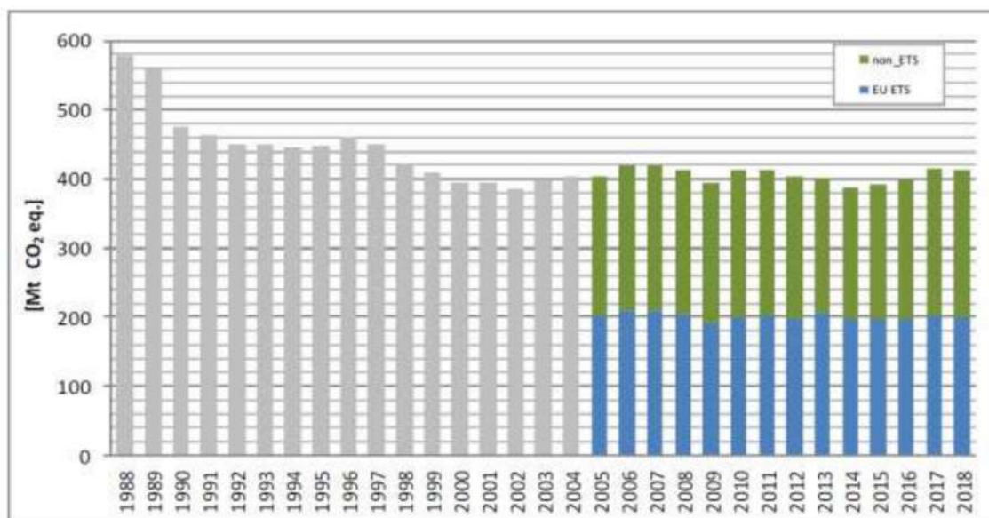
Rysunek 24. Emisja gazów cieplarnianych w Polsce w latach 1988-2018 (bez kategorii LULUCF) 71
