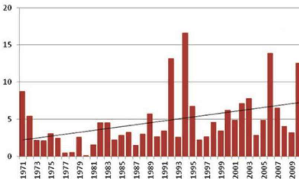
Rysunek 20. Zmienność liczby dni upalnych (temp. max \geq 30^{\circ}\text{C} ) w Polsce w latach 1971-2010 60
