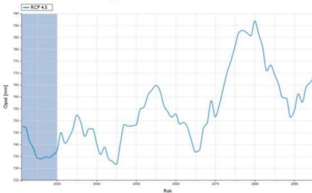
Rysunek 23. Dziesięcioletnia średnia krocząca rocznej sumy opadu dla Polski wg projekcji klimatycznych – scenariusz RCP 4.5 68
