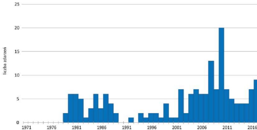
Rysunek 21. Trąby powietrzne w Polsce w latach 1971-2016 62
