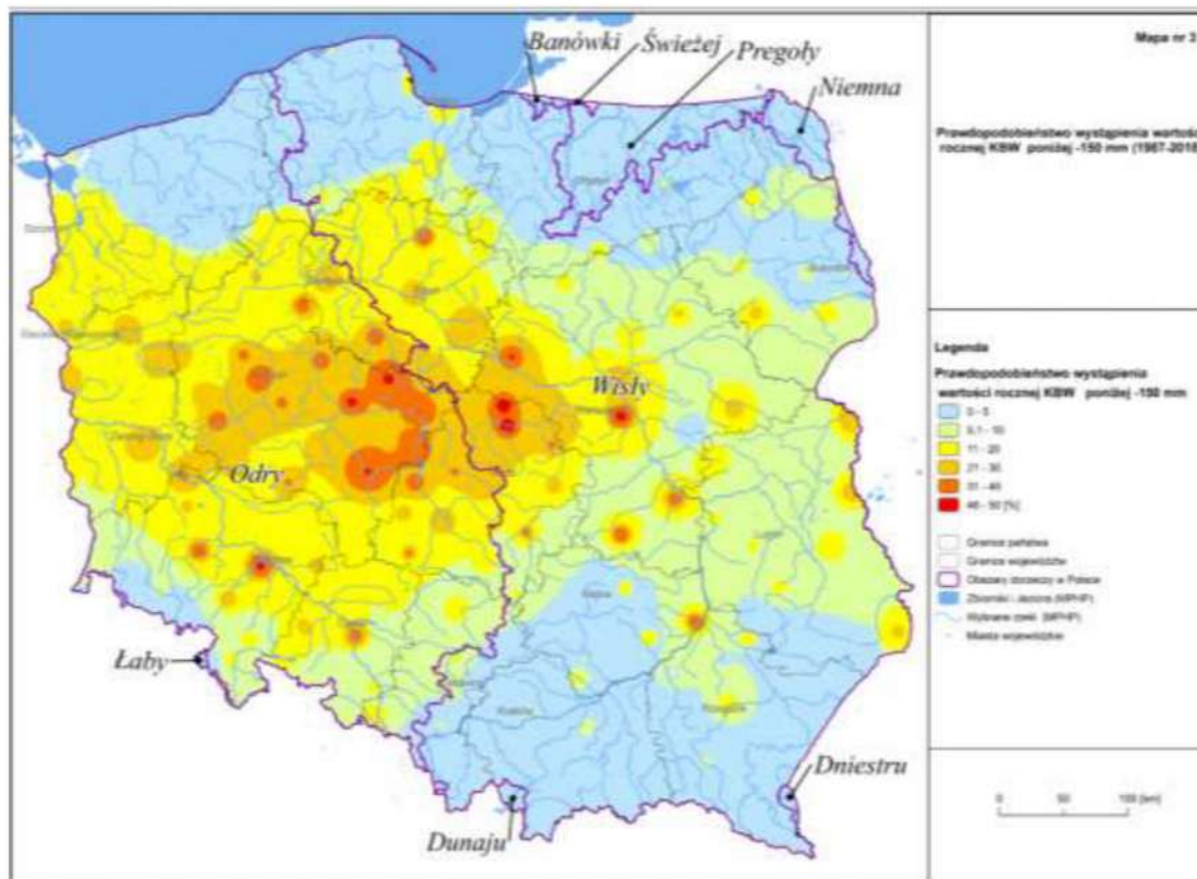
Rysunek 72. Prawdopodobieństwo wystąpienia wartości rocznej Klimatycznego Bilansu Wodnego poniżej wartości -150 \text{ mm}^{162}
