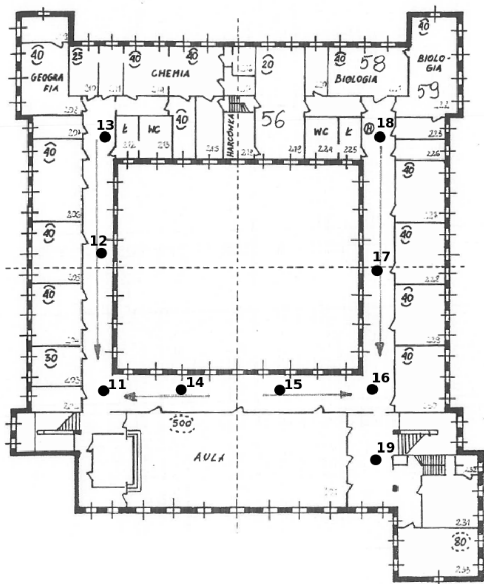
Rys. 1b: Plan rozmieszczenia punktów pomiarowych – I piętro
