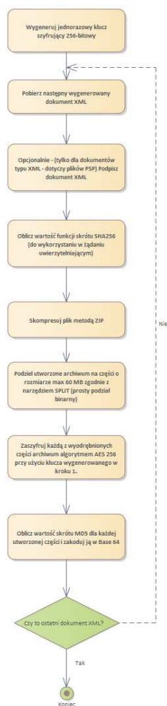
Rysunek: Schemat blokowy kroków przygotowywania do wysyłki danych.
