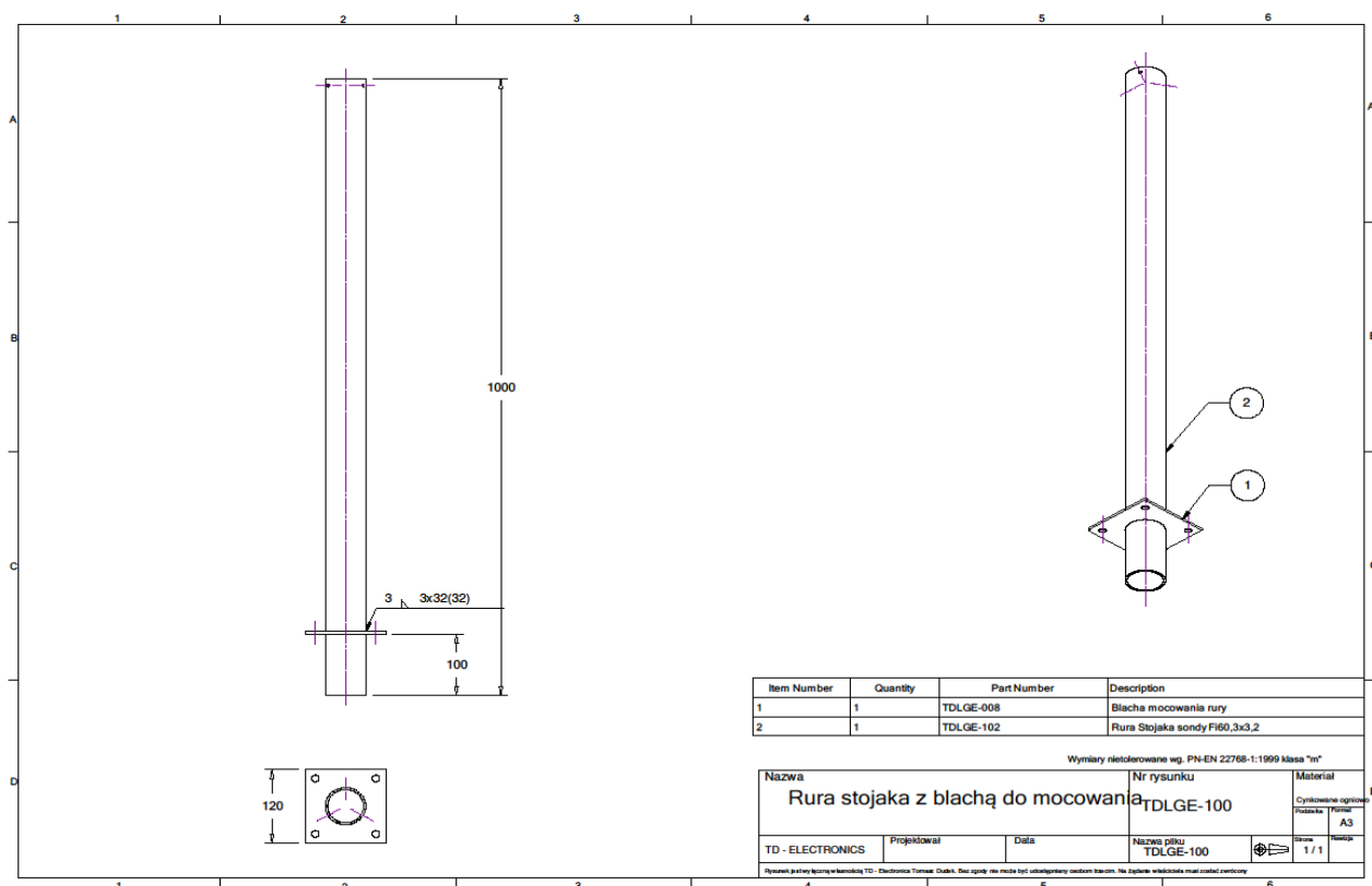
Rys. 2 Stojak sondy.
