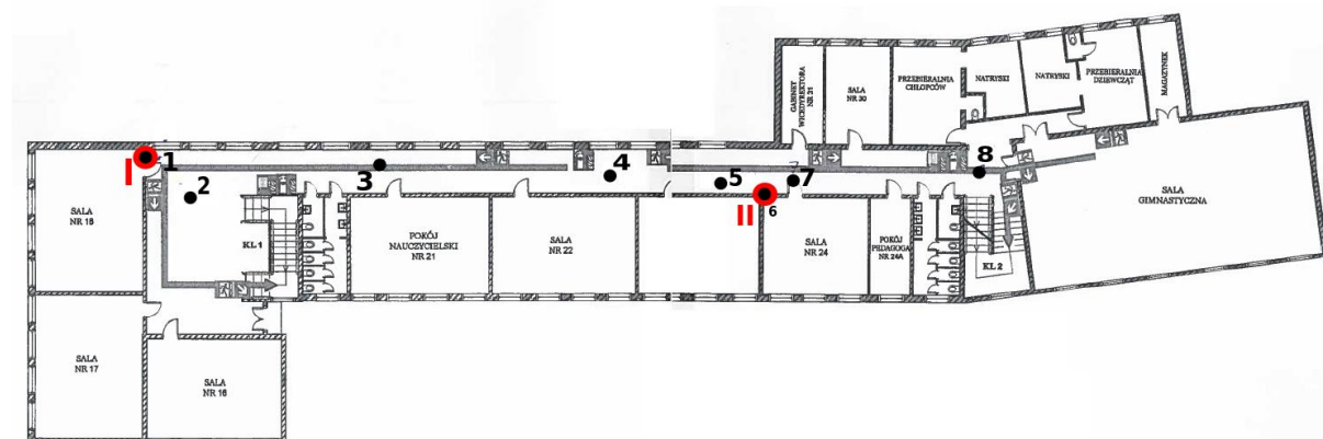
Rys. 1c: Plan rozmieszczenia punktów pomiarowych – I piętro, kolorem czerwonym oznaczono lokalizację punktów dostępowych
