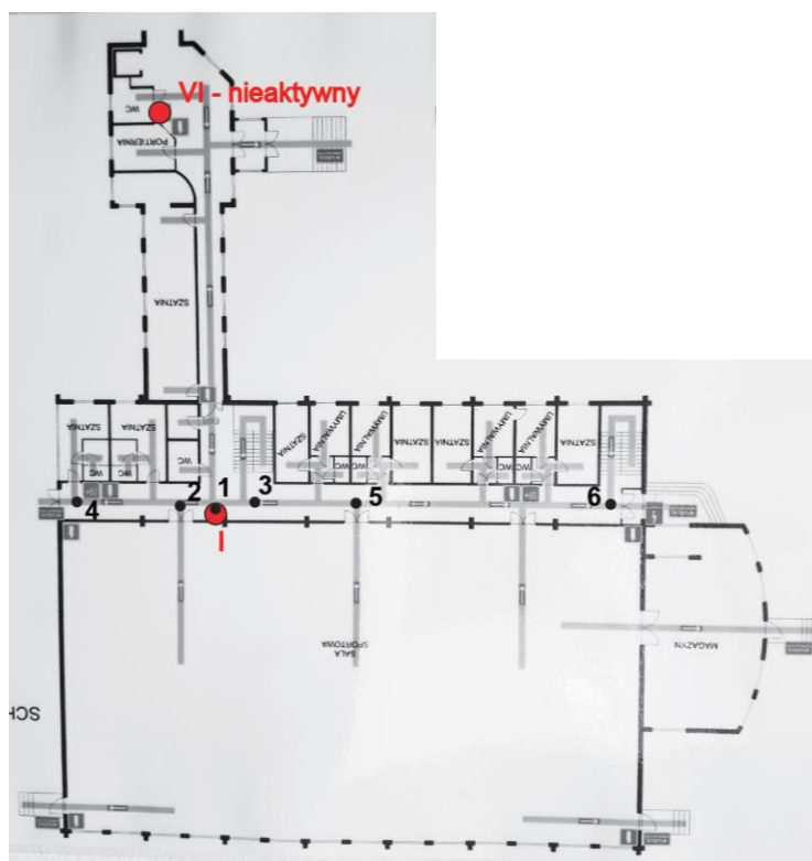
Rys. 1a: Plan rozmieszczenia punktów pomiarowych – parter i przyziemie kolorem czerwonym oznaczono lokalizację punktów dostępowych
