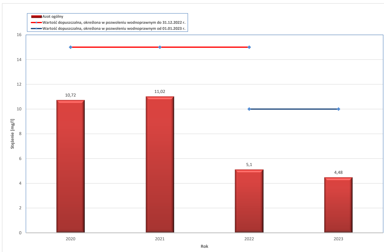
Wykres 7. Średnioroczne stężenie azotu ogólnego w ściekach oczyszczonych w latach 2019 – 2023.
