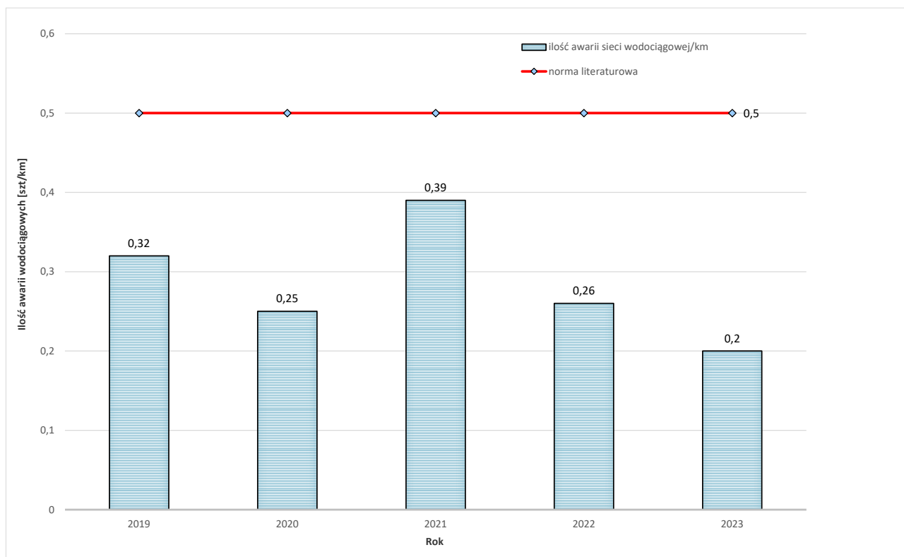
Wykres 4. Awaryjność sieci wodociągowej w latach 2019 – 2023.
