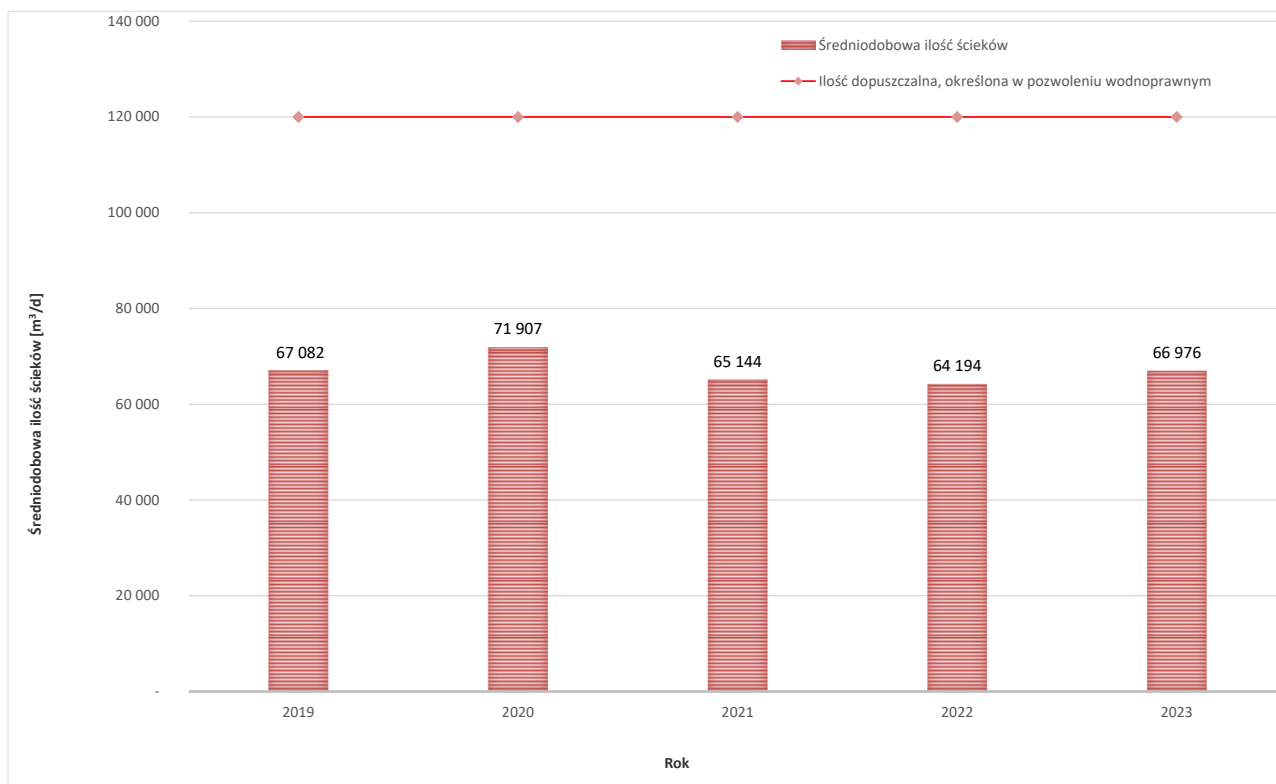
Wykres 6. Średniodobowa ilość ścieków oczyszczonych w Oczyszczalni ścieków „Hajdów” w latach 2019 – 2023.
