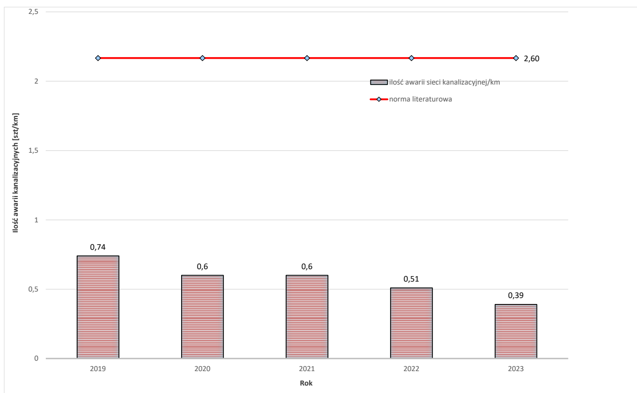
Wykres 5. Awaryjność sieci kanalizacyjnej w latach 2019 – 2023.
