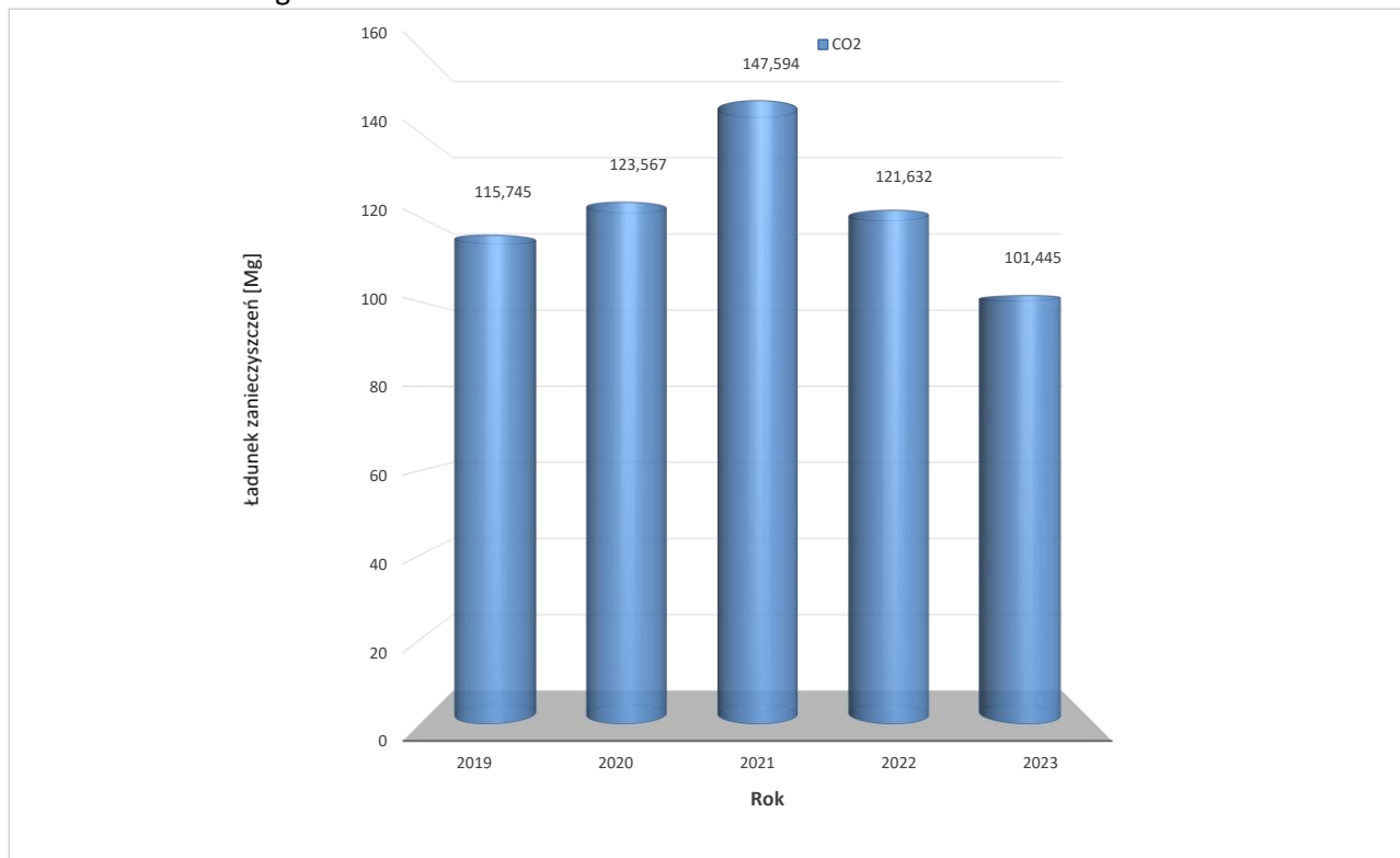
Wykres 16. Zsumowana wielkość emisji CO 2 z lokalnych kotłowni w latach 2019 – 2023.
