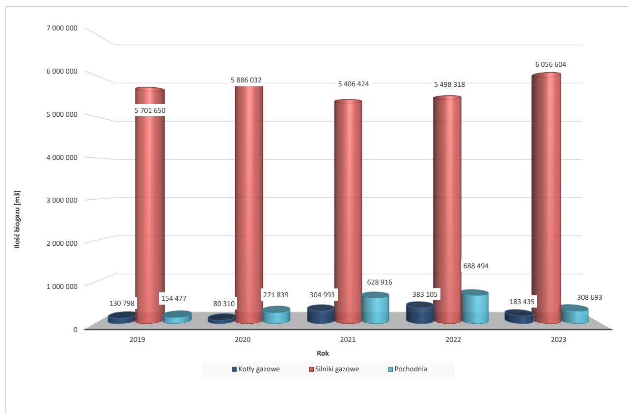
Wykres 20. Wykorzystanie biogazu na Oczyszczalni Ścieków „Hajdów” w latach 2019 – 2023.
