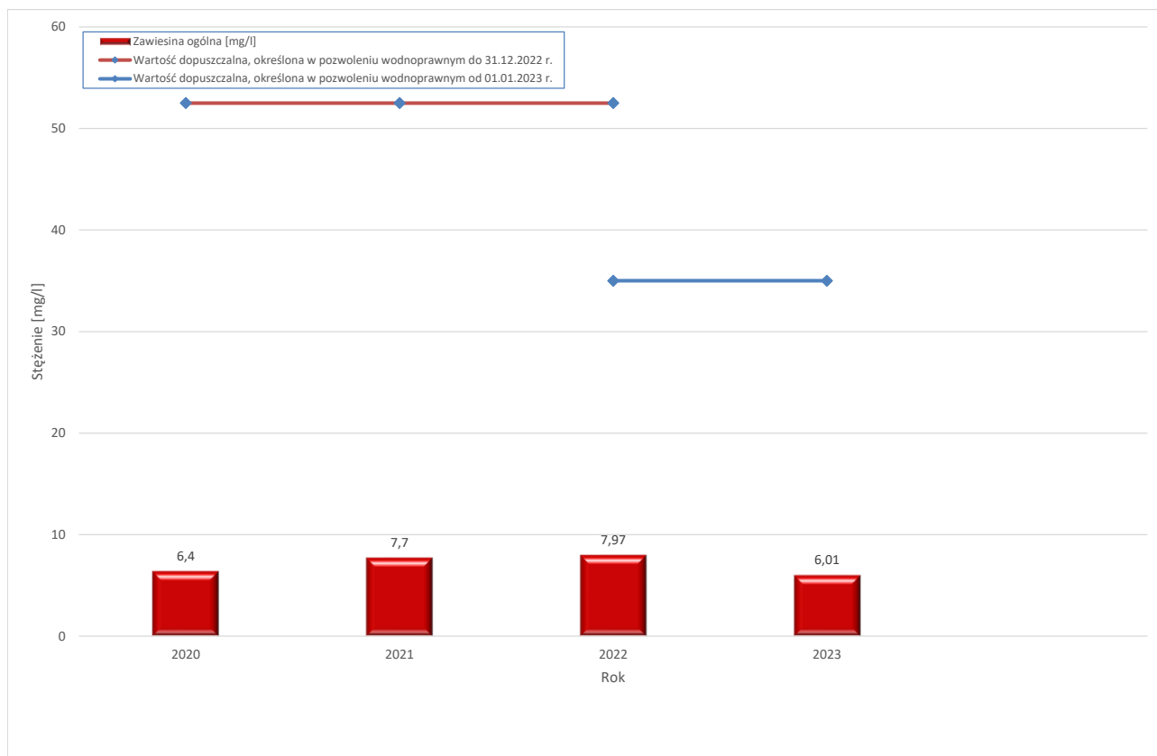
Wykres 11. Średnioroczne stężenie zawiesiny ogólnej w ściekach oczyszczonych w latach 2019 – 2023.
