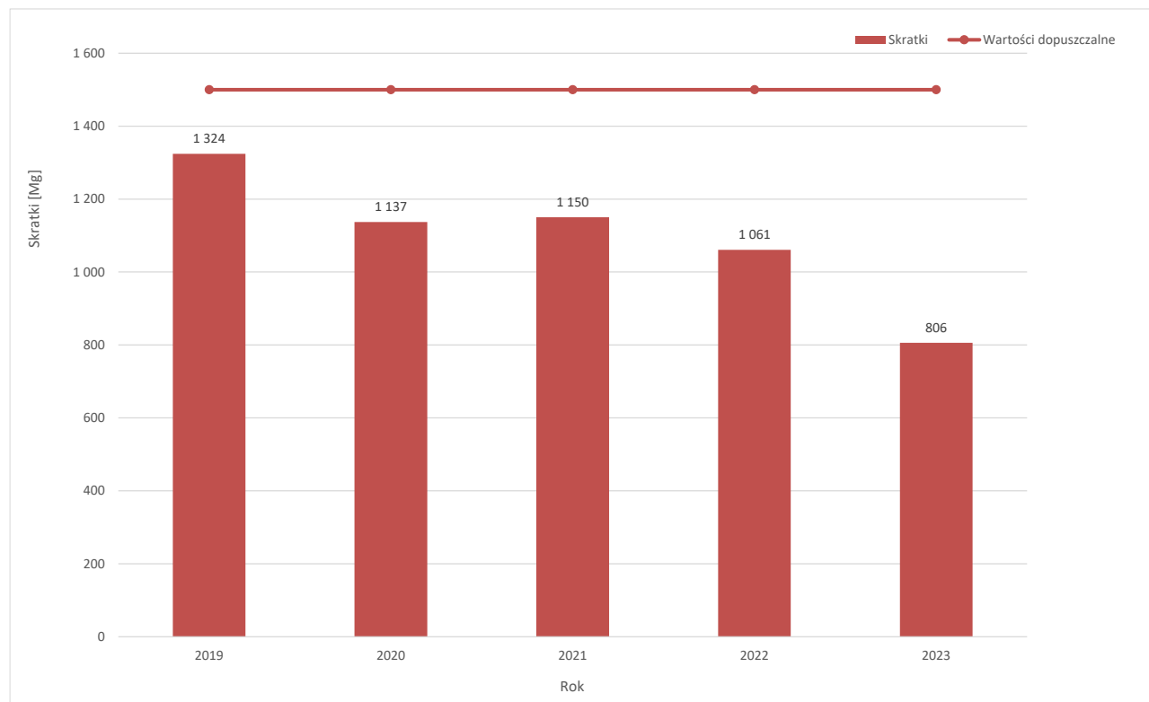
Wykres 12. Ilość skratek wytworzonych w latach 2019 – 2023.
