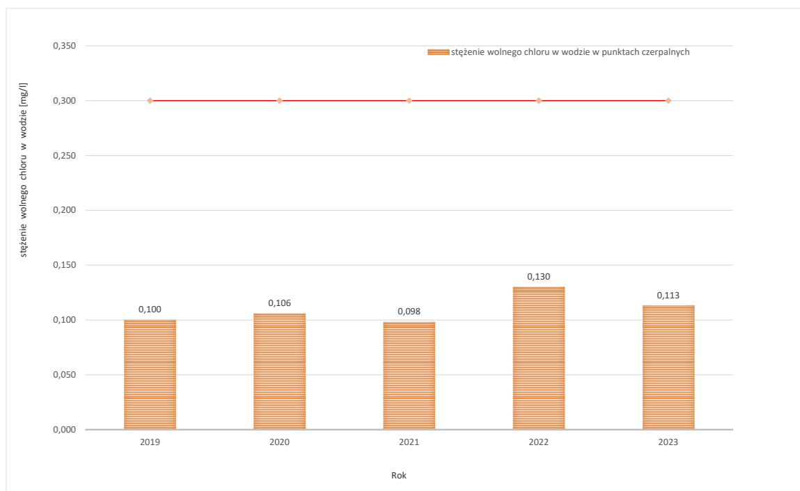
Wykres 2. Średnioroczne stężenia wolnego chloru w wodzie w punktach czerpalnych w odniesieniu do wartości określonych w rozporządzeniu w latach 2019 – 2023.
