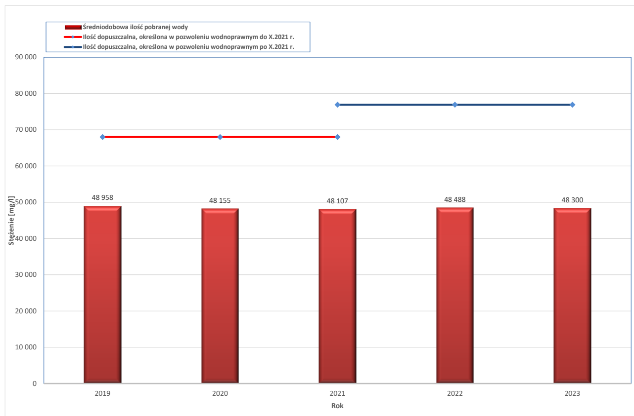
Wykres 3. Średniobodobowa ilość pobranej wody w latach 2019 – 2023.
