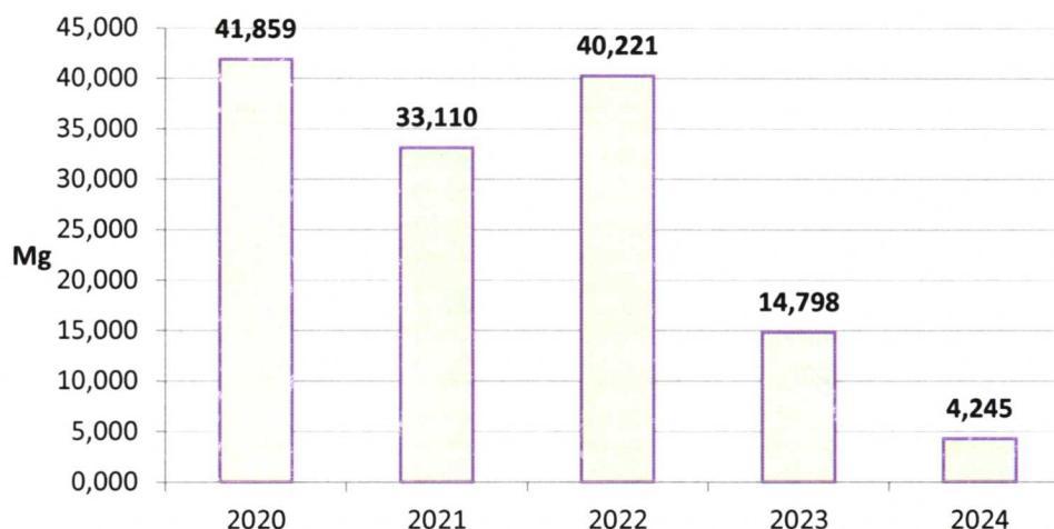
Zużycie koagulantu w Mg w przeliczeniu na 1 mln m 3 ścieków
