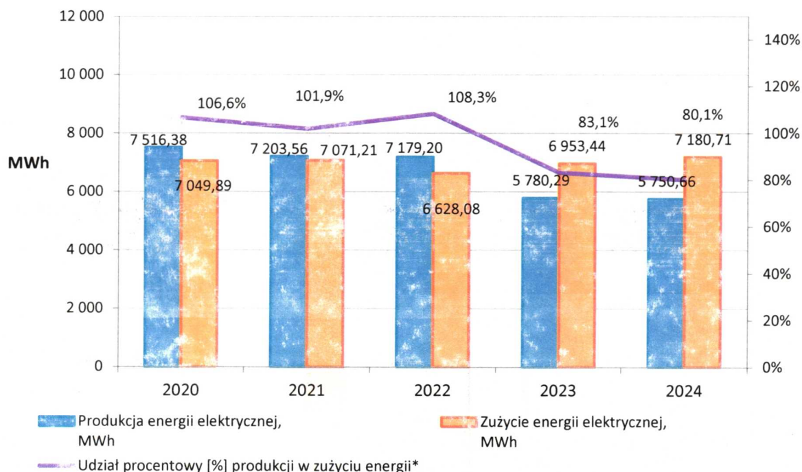
Bilans energii elektrycznej RCGW S.A w MWh/rok
