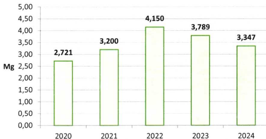
Zużycie flokulantu na Stacji odwadniania w Mg w przeliczeniu na 1 mln m3 ścieków
