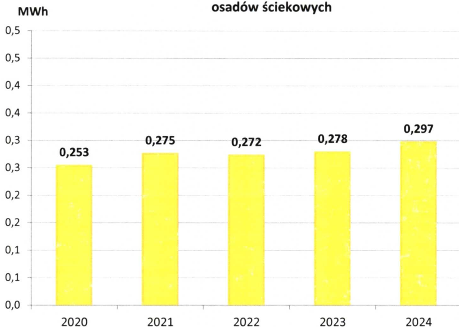
Ilość zużytej energii elektrycznej w MWh na 1Mg wytworzonych osadów ściekowych
