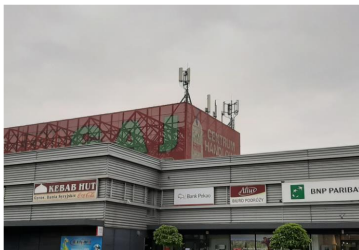
Fot. 1: Widok anten stacji bazowych: ID: BT34229, ID: 14246 oraz ID: WRO1112, zlokalizowanych przy ul. Świeradowskiej 51-57 we Wrocławiu
