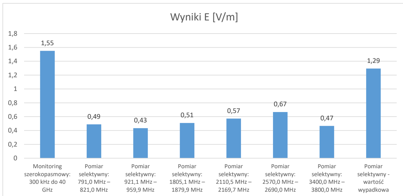
Rys. 17 Porównanie wyników monitoringu szerokopasmowego i pomiarów selektywnych
