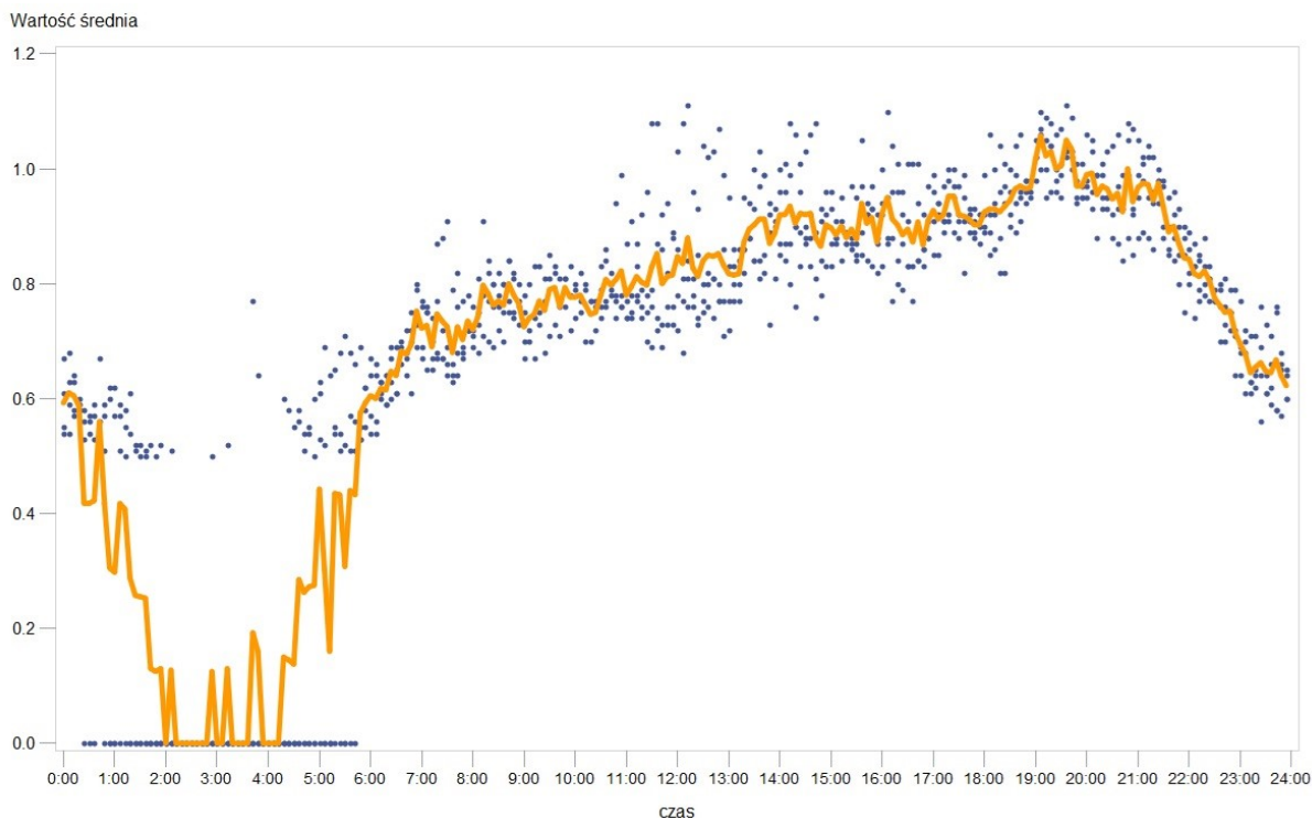
Rys. 9 Wyniki pomiarów – Przedszkole nr 20 w Piotrkowie Trybunalskim – średnia za okres 24 godzin
