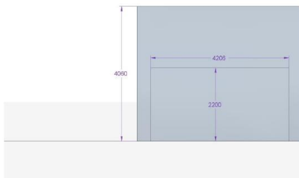
Szkic 6 Zabudowa front
