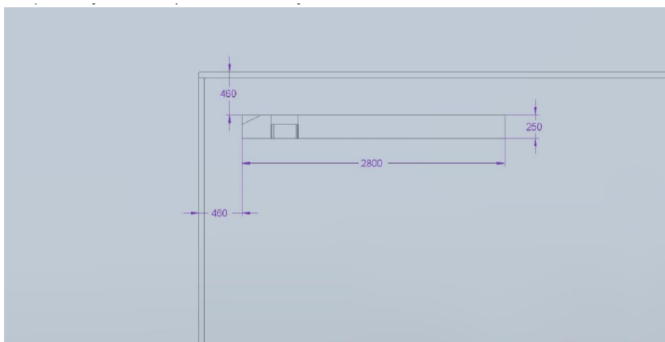
Szkic 8 Sufit. Otwór wentylacyjny
