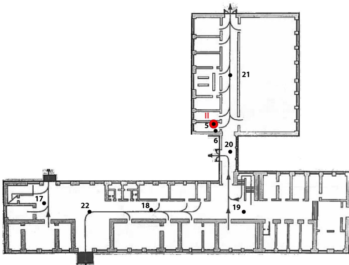
Rys. 1a: Plan rozmieszczenia punktów pomiarowych – parter, kolorem czerwonym oznaczono lokalizację punktu dostępowego
