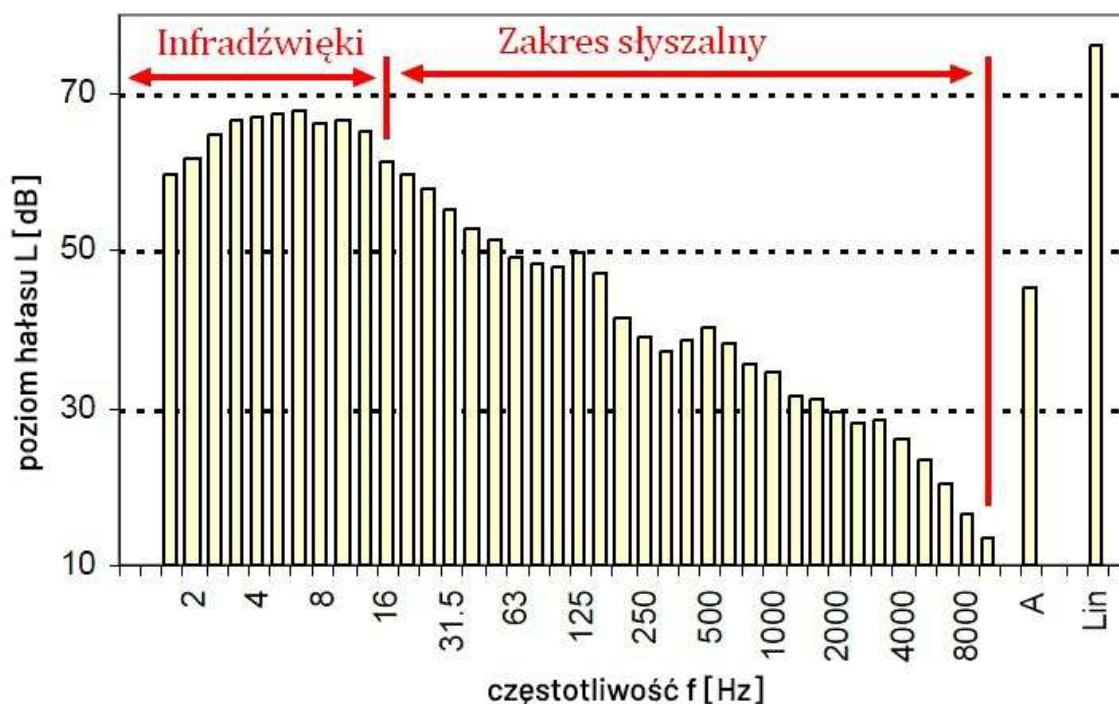
Rys. 1.8. Widmo dźwięku Turbiny Vestas V-80 33 , ze zmianami autora
