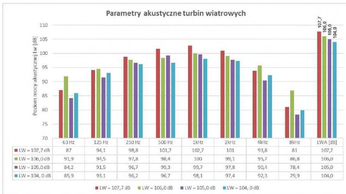
Rys. 1.9. Parametry akustyczne analizowanych turbin wiatrowych
