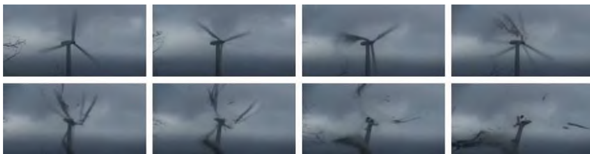
Rys. 1.36. Przypadek awarii katastrofalnej turbiny, możliwa jest obserwacja torów lotu fragmentów łopat (fragmenty materiału 211 )
