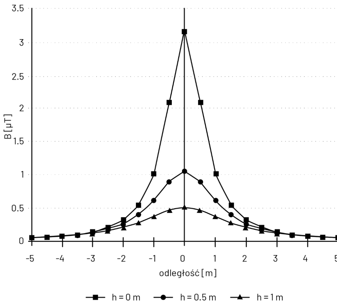
Rys. 1.22. Rozkłady indukcji magnetycznej w odległości od osi linii kablowej 20 kV, która płynie prąd 160 A (indukcja 3,5 \mu\text{T} odpowiada natężeniu pola magnetycznego 2,8 \text{ A/m} ) wg 141
