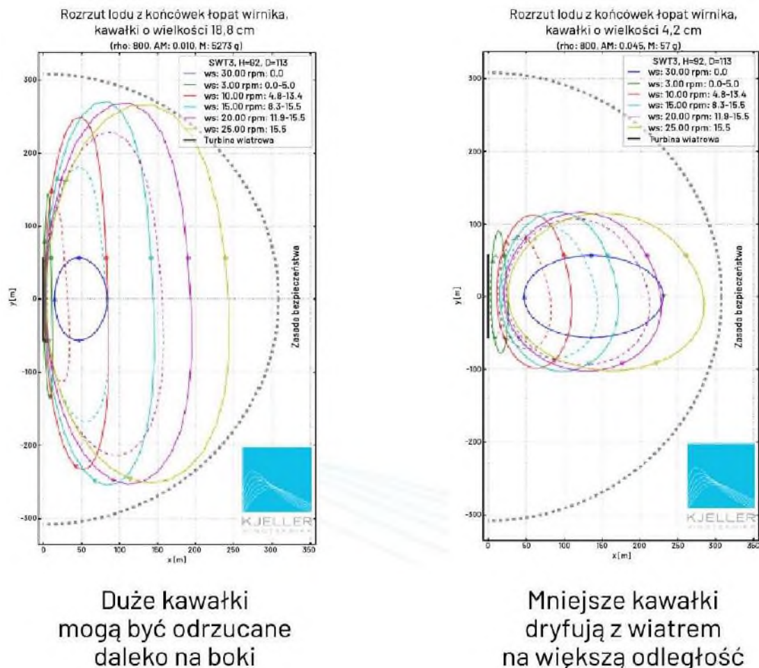
Rys. 1.31. Odległości rzutu odłamków lodowych dla różnych prędkości wiatru (zasięgi zawierają się wewnątrz koła o promieniu 330 m) 174 .
