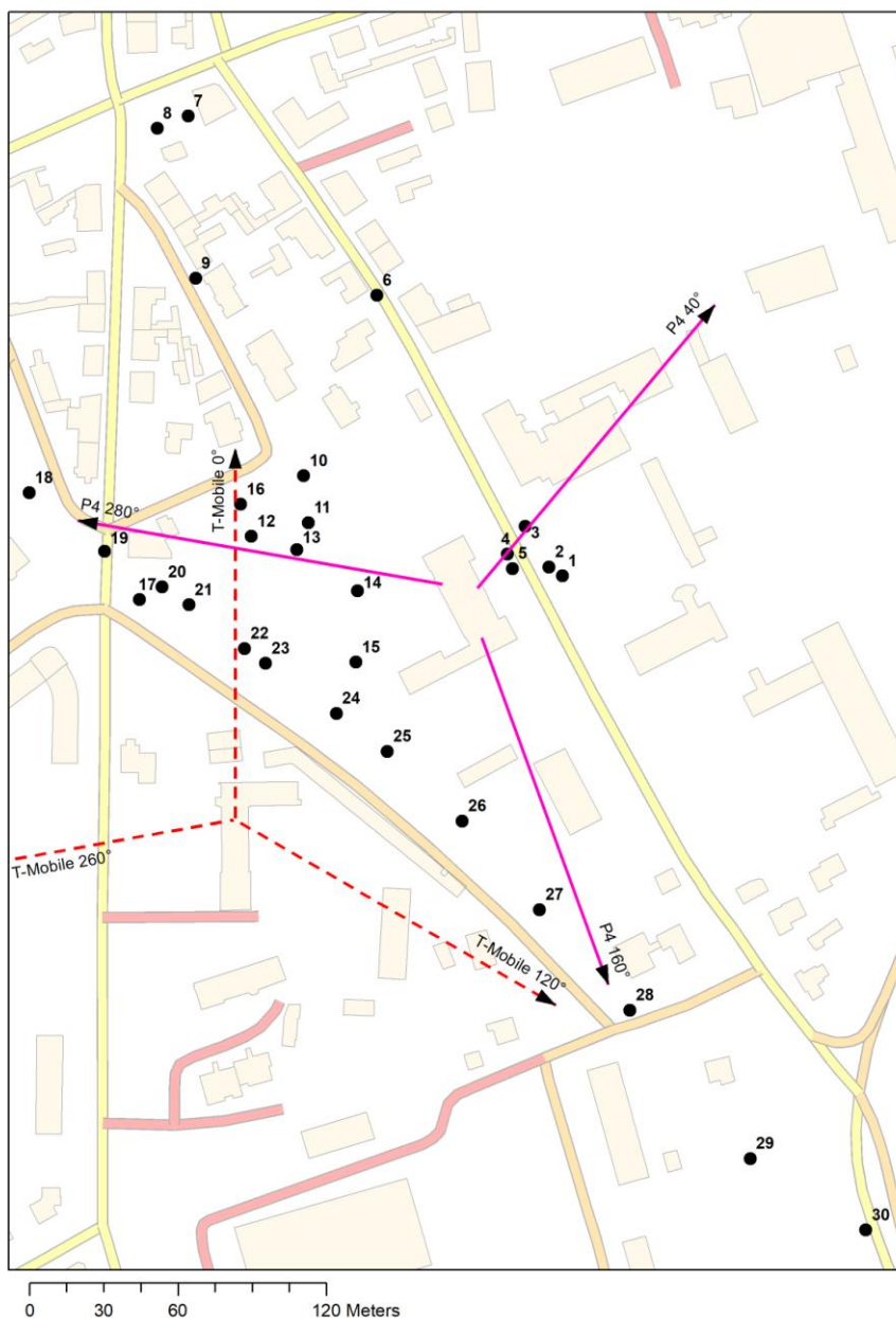
Rys. 1: Plan terenu, na którym znajdują się badana stacja bazowa
