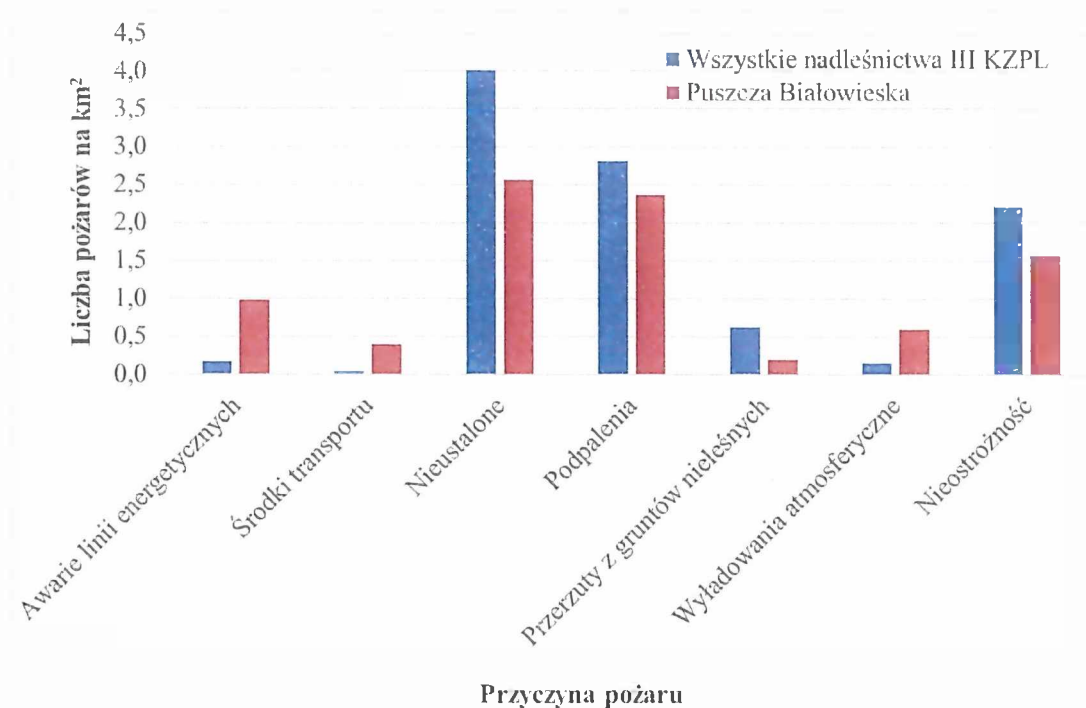
Rycina 2 Rozkład gęstości pożarów lasu w Puszczy Białowieskiej w latach 2007-2019 według przyczyn.
