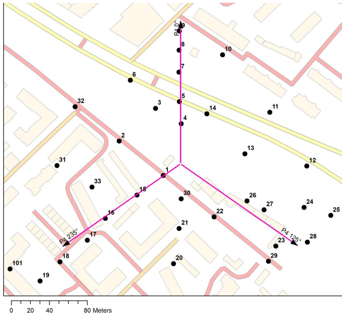
Rys. 1: Plan terenu, na którym znajduje się badana stacja bazowa
