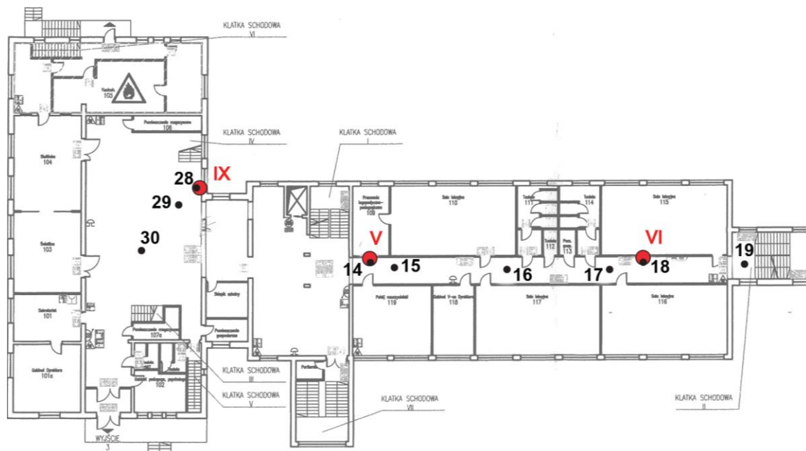
Rys. 1b: Plan rozmieszczenia punktów pomiarowych – parter kolorem czerwonym oznaczono lokalizację punktów dostępnych
