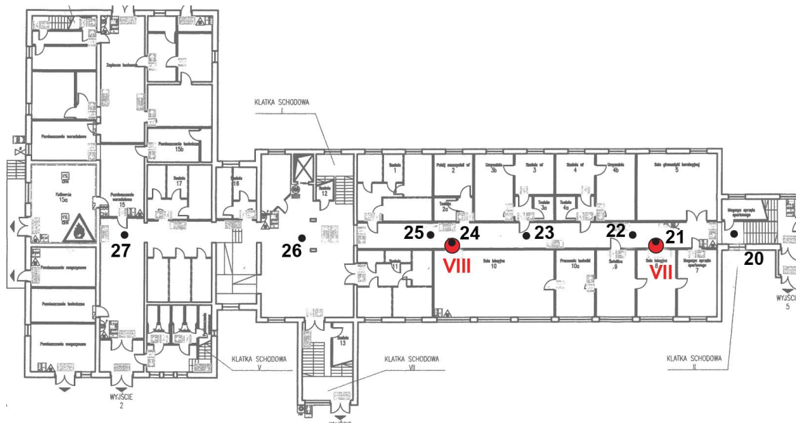
Rys. 1a: Plan rozmieszczenia punktów pomiarowych – przyziemie kolorem czerwonym oznaczono lokalizację punktów dostępnych
