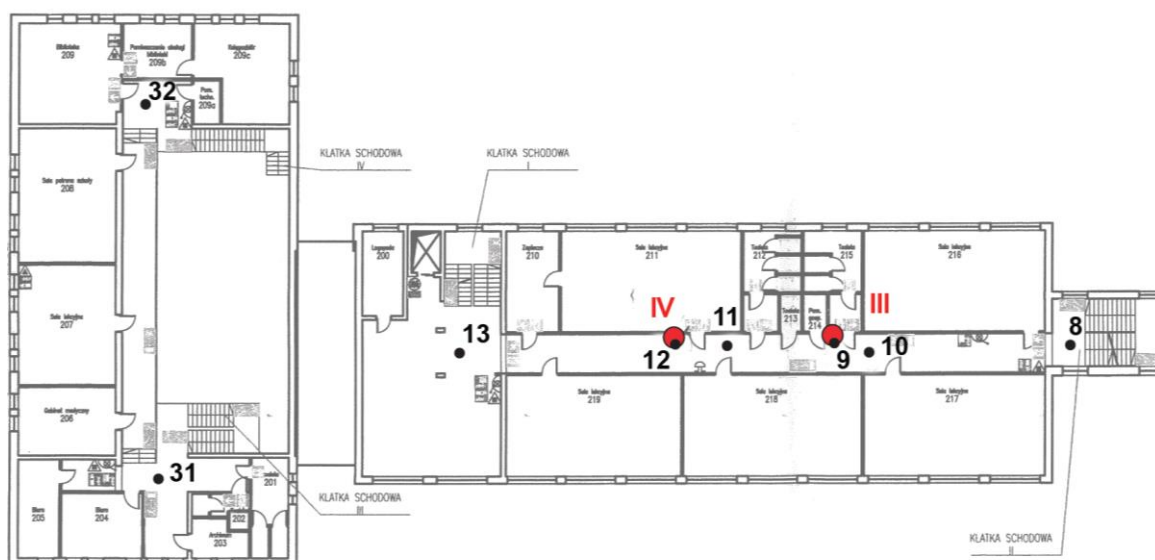
Rys. 1c: Plan rozmieszczenia punktów pomiarowych – I piętro kolorem czerwonym oznaczono lokalizację punktów dostępowych
