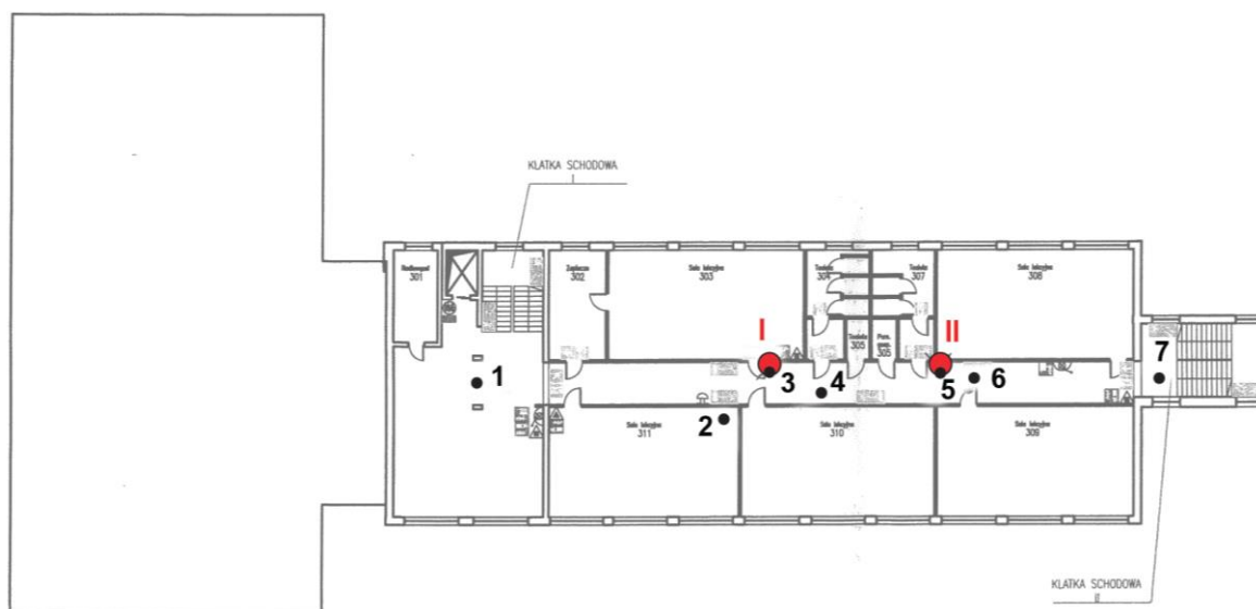
Rys. 1d: Plan rozmieszczenia punktów pomiarowych – II piętro kolorem czerwonym oznaczono lokalizację punktów dostępowych
