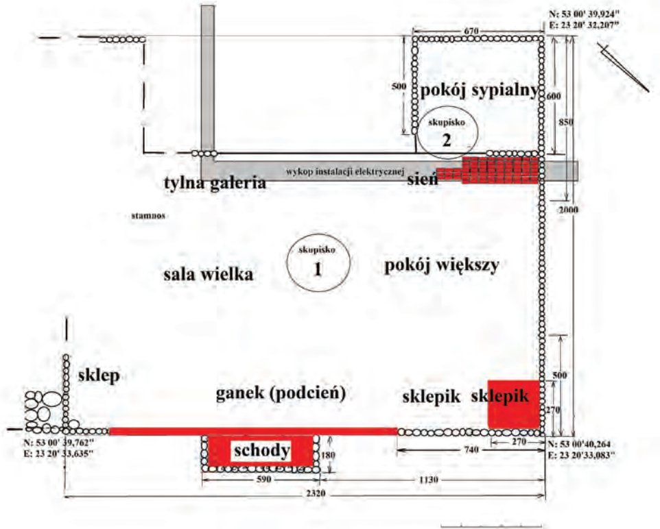
10. Zabłudów. Rekonstrukcja rozplanowania budynku dworskiego z 1622 r. Rys. L. Pawlata Zabłudów. Reconstruction of the manor building layout from 1622. Sketch by L. Pawlata
