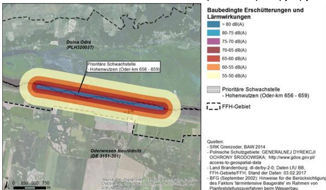
Rys. 5: Przedziały imisji hałasu na przykładzie priorytetowego miejsca limitującego Hohenwutzen (kilometr 656 - 659).
