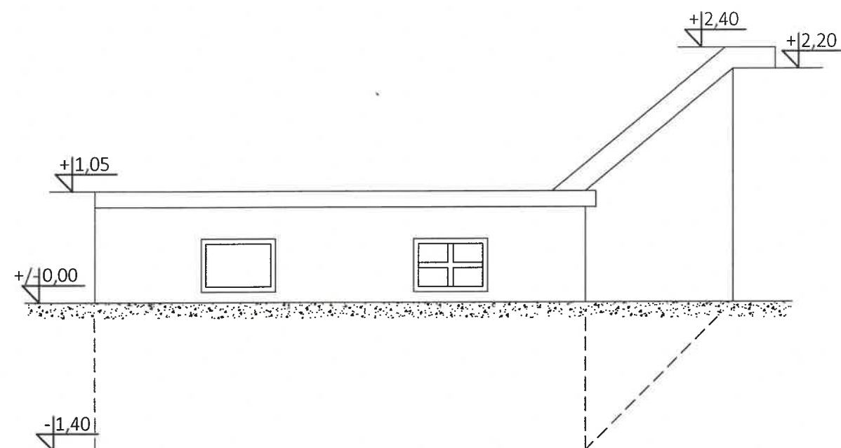
ELEWACJA PÓŁNOCNO-ZACHODNIA
