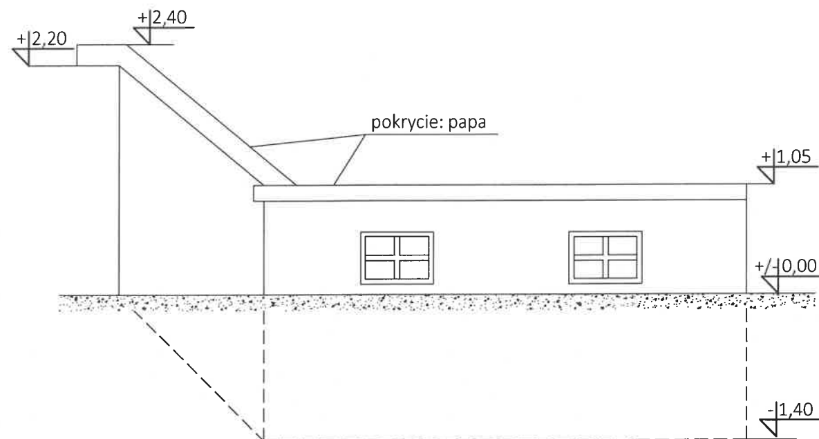
ELEWACJA POŁUDNIOWO-WSCHODNIA
