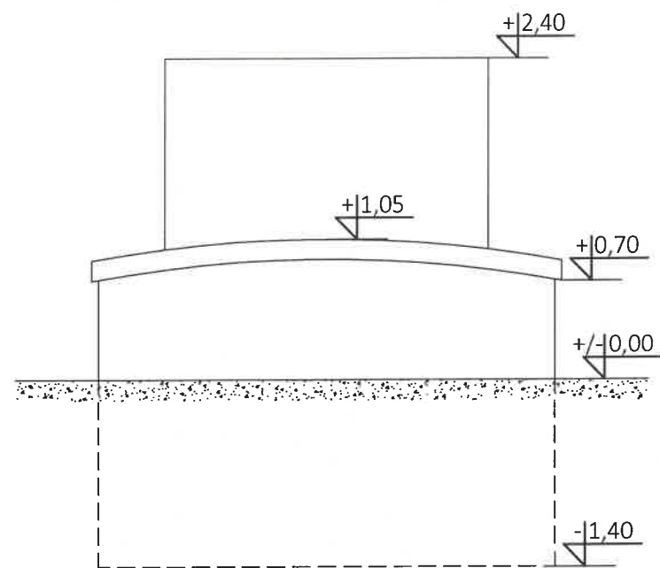
ELEWACJA PÓŁNOCNO-WSCHODNIA
