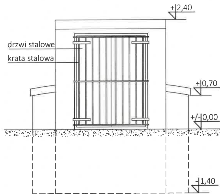
ELEWACJA POŁUDNIOWO-ZACHODNIA
