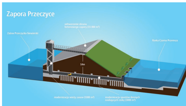
Ryc. 1. Poglądowy zakres prac modernizacyjnych
