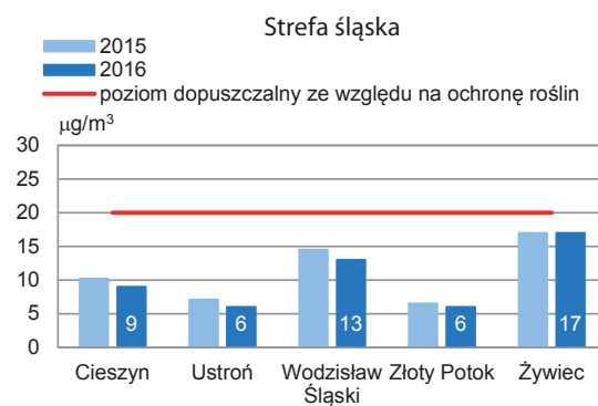
Wykres 12. Stężenia średnie roczne dwutlenku siarki w latach 2015-2016 w miastach i aglomeracjach oraz strefie śląskiej
