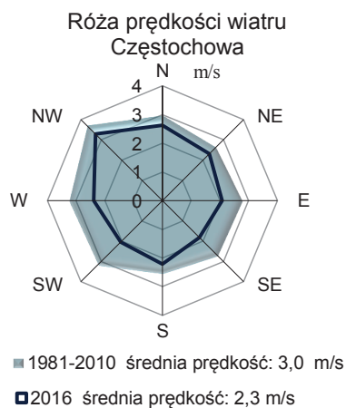
Wykres 23. Róże wiatru dla stacji meteorologicznych PSHM IMGW-PIB w województwie śląskim w roku 2016 na tle okresu wieloletniego 1981-2010
