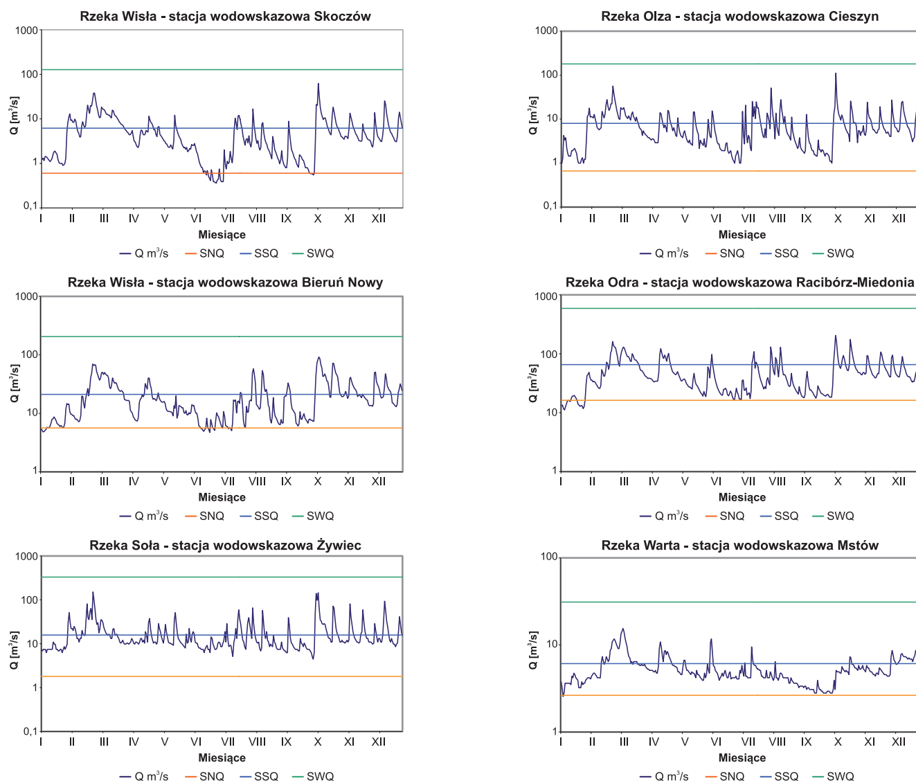
Wykres 8. Hydrogramy przepływów w 2016 roku dla wybranych stacji wodowskazowych
