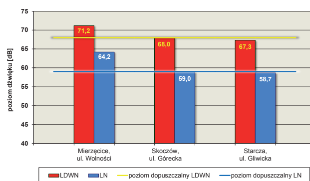
Wykres 6. Wielkości średniorocznych wskaźników oceny hałasu L_{DWN} i L_N dla wyszczególnionych miejscowości objętych monitoringiem hałasu drogowego w 2016 r.
