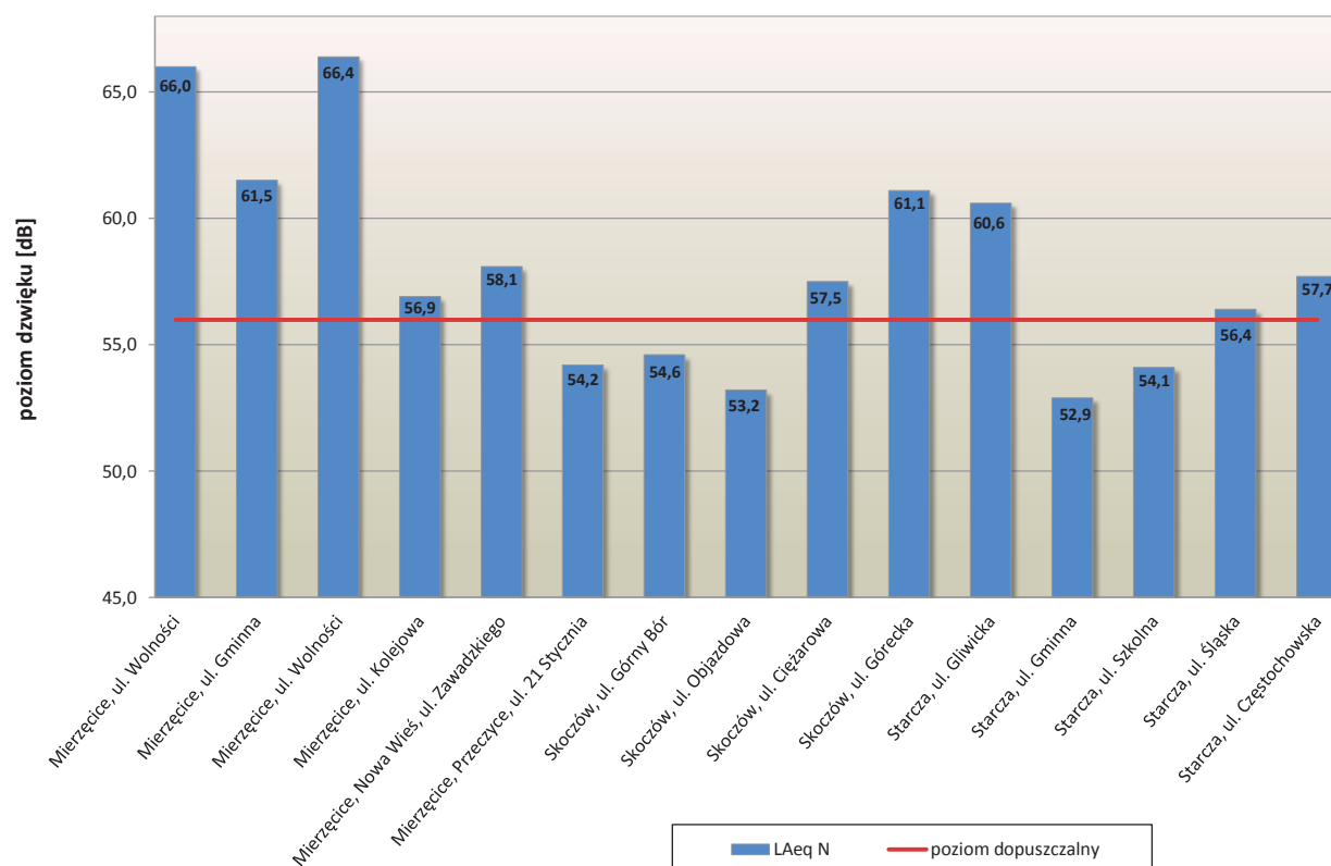
Wykres 8. Wielkości krótkookresowych wskaźników oceny hałasu L_{Aeq N} dla wymienionych miejscowości objętych monitoringiem hałasu drogowego w 2016 r.
