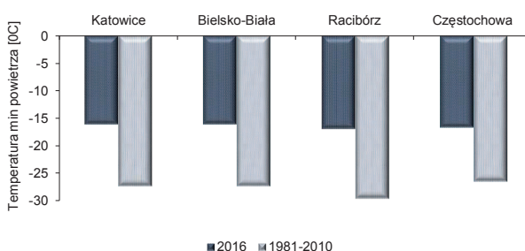
Wykres 19. Średnia roczna, maksymalna (max) i minimalna (min) temperatura powietrza dla stacji meteorologicznych PSHM IMGW-PIB w województwie śląskim w roku 2016 na tle okresu wieloletniego 1981-2010
