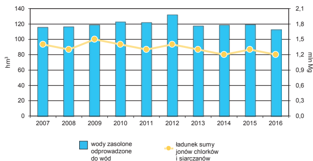
Wykres 4. Ilość wód zasolonych i ładunek sumy jonów chlorków ( \text{Cl}^- ) i siarczanów ( \text{SO}_4^{2-} ) odprowadzonych do wód w latach 2007-2016
