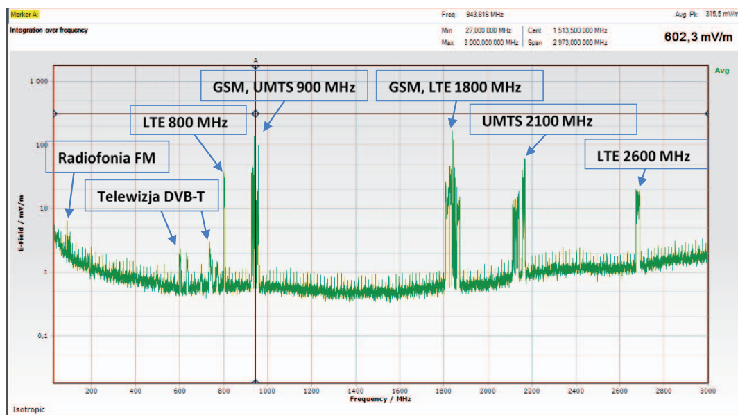
Ryc. 1. Widmo pola elektromagnetycznego z opisem źródeł – punkt pomiarowy w Chybiu przy ul. Kolejowej
