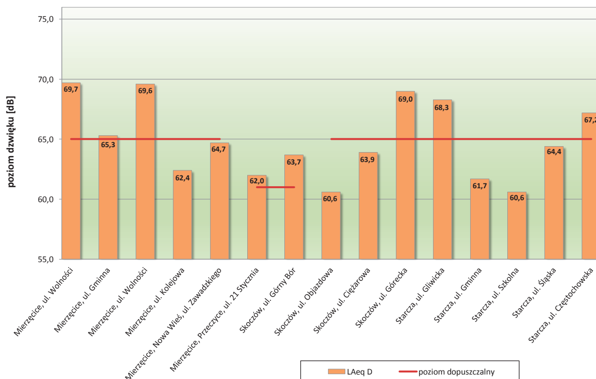
Wykres 7. Wielkości krótkookresowych wskaźników oceny hałasu L_{Aeq D} dla wymienionych miejscowości objętych monitoringiem hałasu drogowego w 2016 r.
