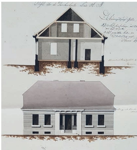
9. Projekt domu mieszkalnego dla inspektora Himmel w Bielsku, 1805 r., APB, Kamera Wojny i Domen, sygn. 2830, k. 406 Residential building design for Inspector Himmel in Bielsk, 1805, State Archive in Białystok, War and Domain Office, ref. 2830, k. 406
