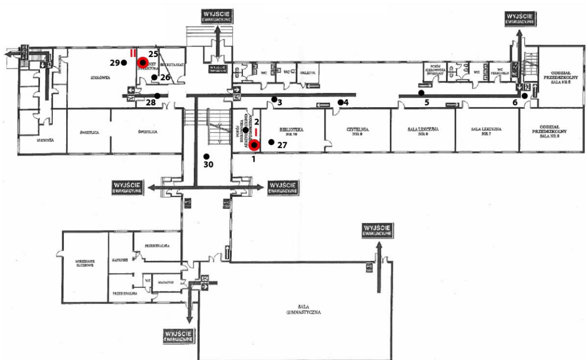
Rys. 1b: Plan rozmieszczenia punktów pomiarowych – parter, kolorem czerwonym oznaczono lokalizację punktów dostępowych
