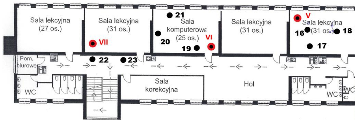
Rys. 1d: Plan rozmieszczenia punktów pomiarowych – piętro, część 2 kolorem czerwonym oznaczono lokalizację punktów dostępowych
