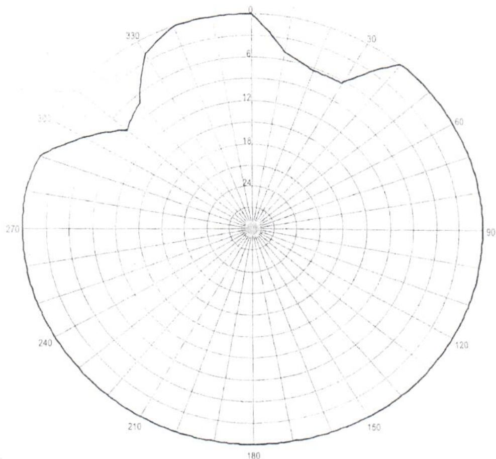
Pozioma charakterystyka promieniowania anteny stacji Płock 88,10 MHz
