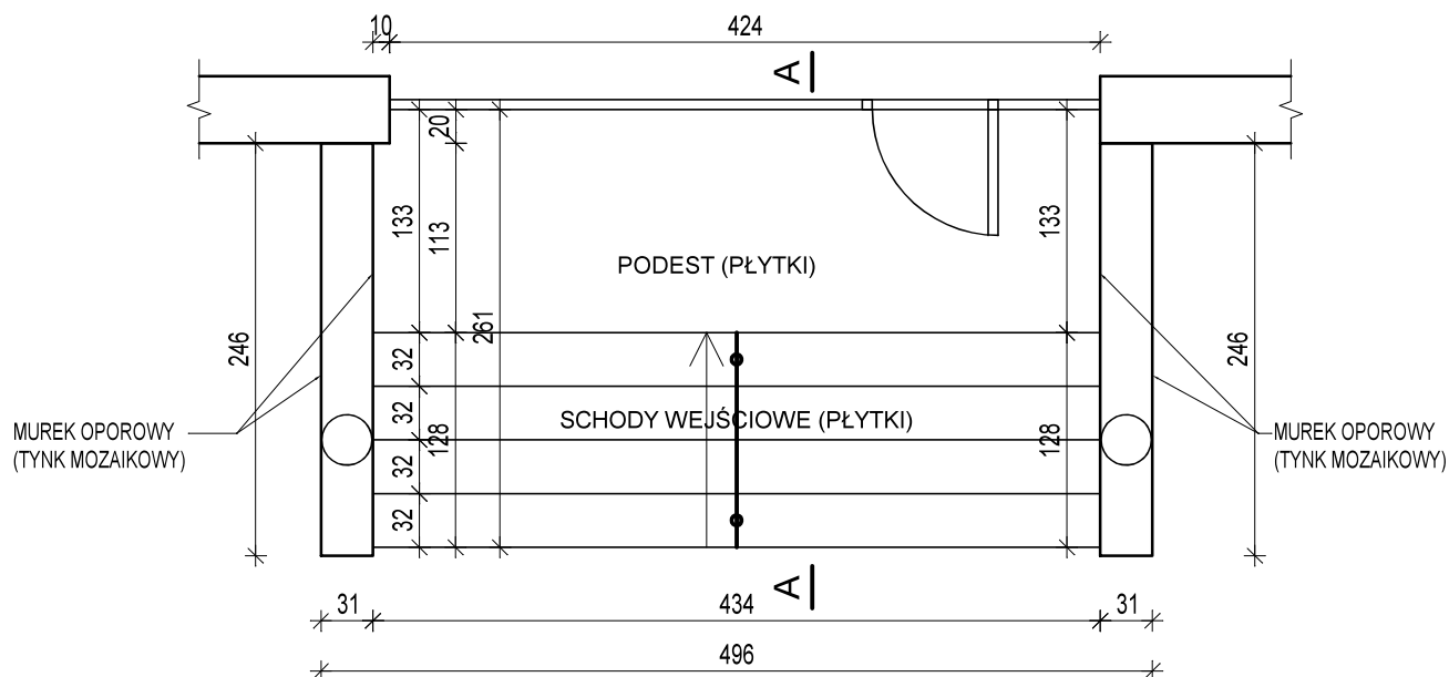
RZUT SCHODÓW
