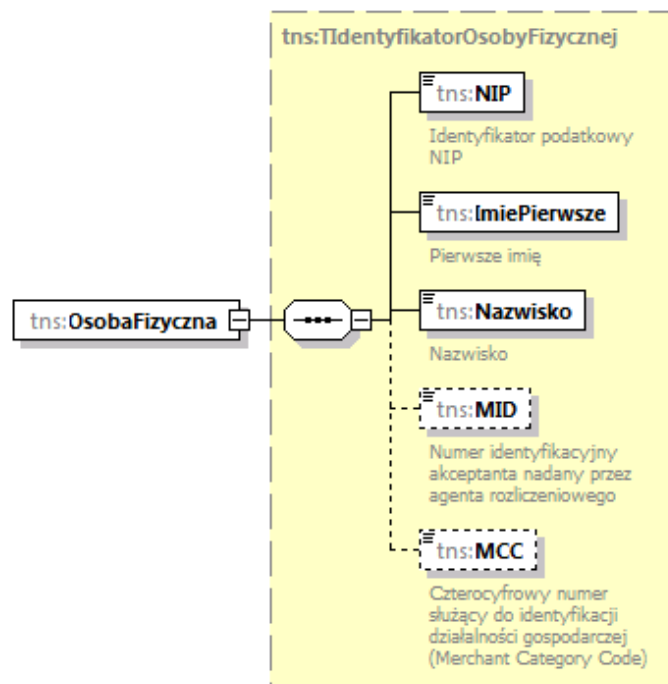
Schemat 10. Struktura danych identyfikujących Akceptanta będącego osobą fizyczną w ITP.
