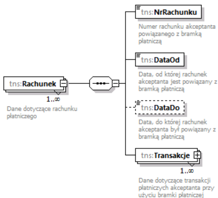
Schemat 18. Struktura danych dotyczących rachunku akceptanta powiązanego z bramką płatniczą w ITP.
