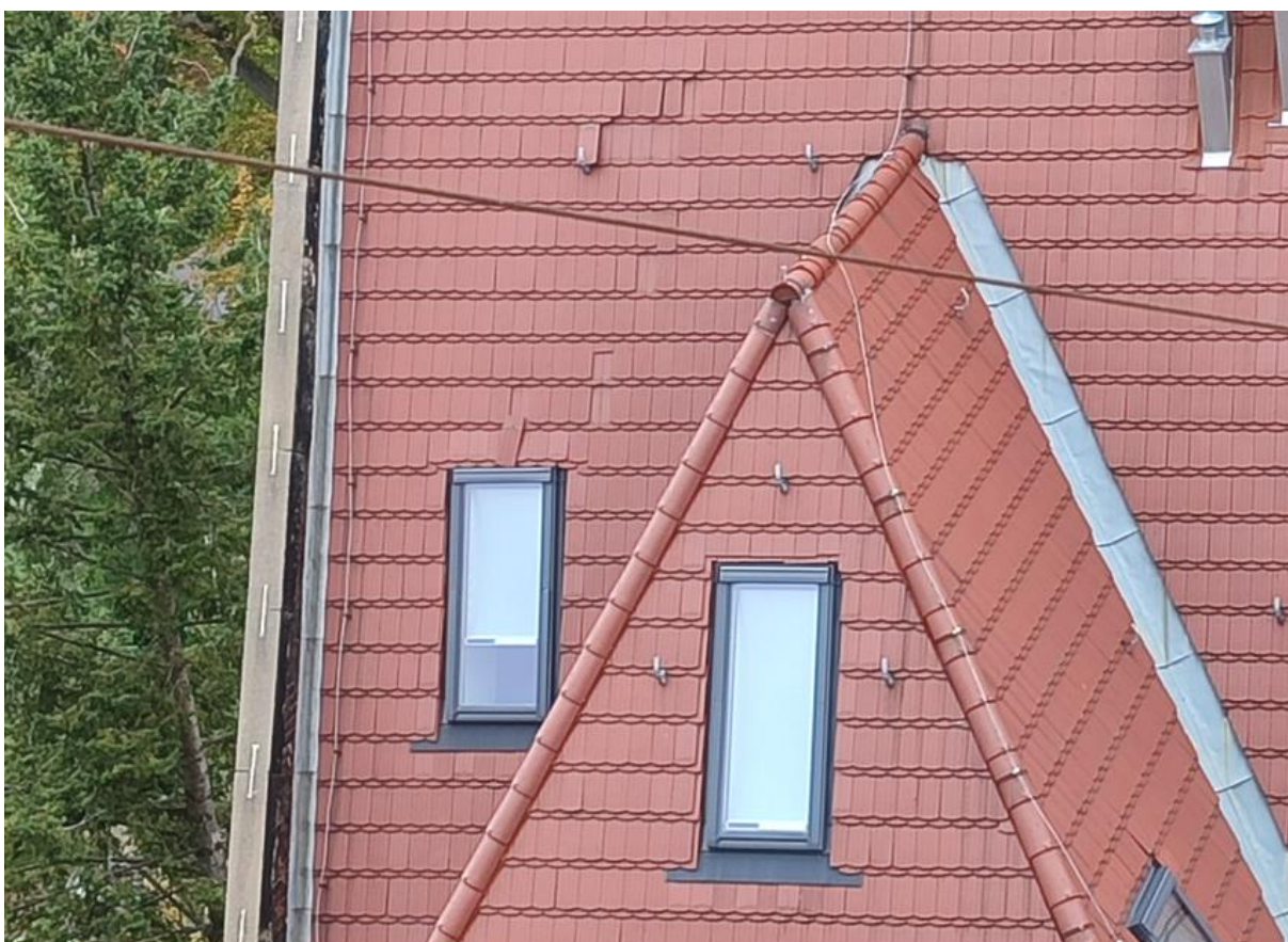
Uszkodzony kosz zlewowy i oderwane dachówki w obrębie kosza.
