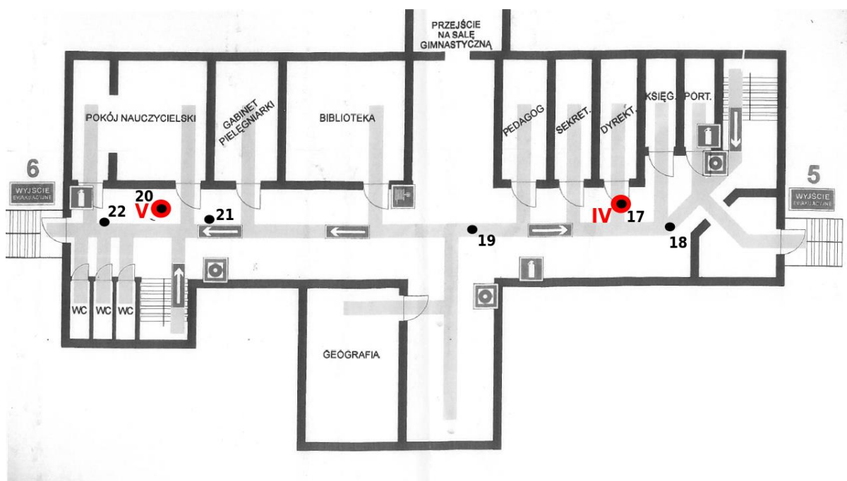
Rys. 1b: Plan rozmieszczenia punktów pomiarowych – parter, część B, kolorem czerwonym oznaczono lokalizację punktów dostępnych.
