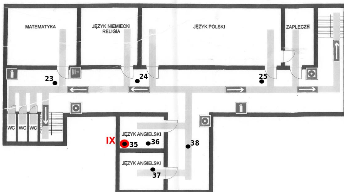
Rys. 1c: Plan rozmieszczenia punktów pomiarowych – I piętro, część A.
