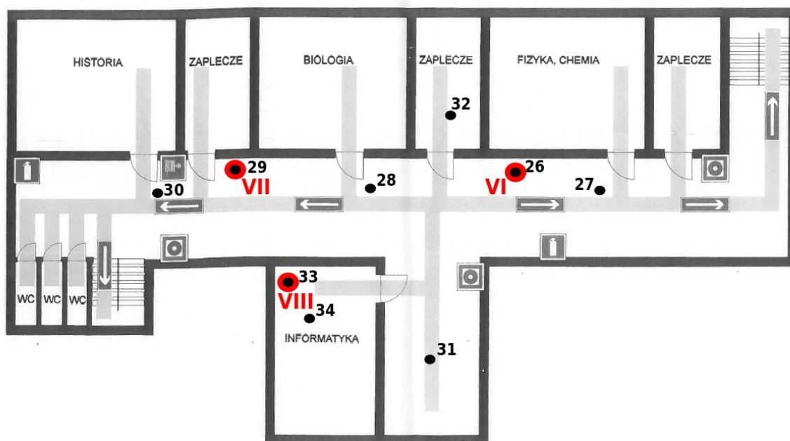
Rys. 1f: Plan rozmieszczenia punktów pomiarowych – II piętro, część B, kolorem czerwonym oznaczono lokalizację punktów dostępowych
