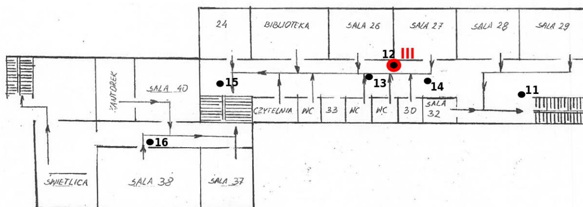
Rys. 1e: Plan rozmieszczenia punktów pomiarowych – II piętro, część A, kolorem czerwonym oznaczono lokalizację punktów dostępowych
