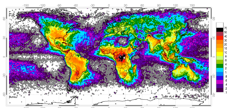
Rys. 1. Natężenie występowania wyładowań piorunowych na powierzchni 1 km 2 w ciągu roku [3]
