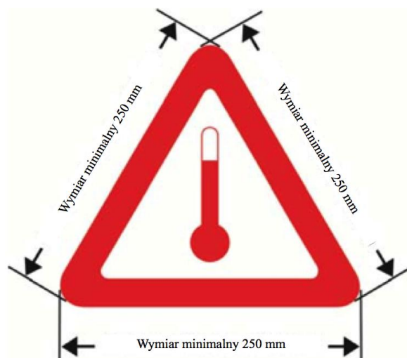
Znak dla przewozu materiałów o podwyższonej temperaturze
