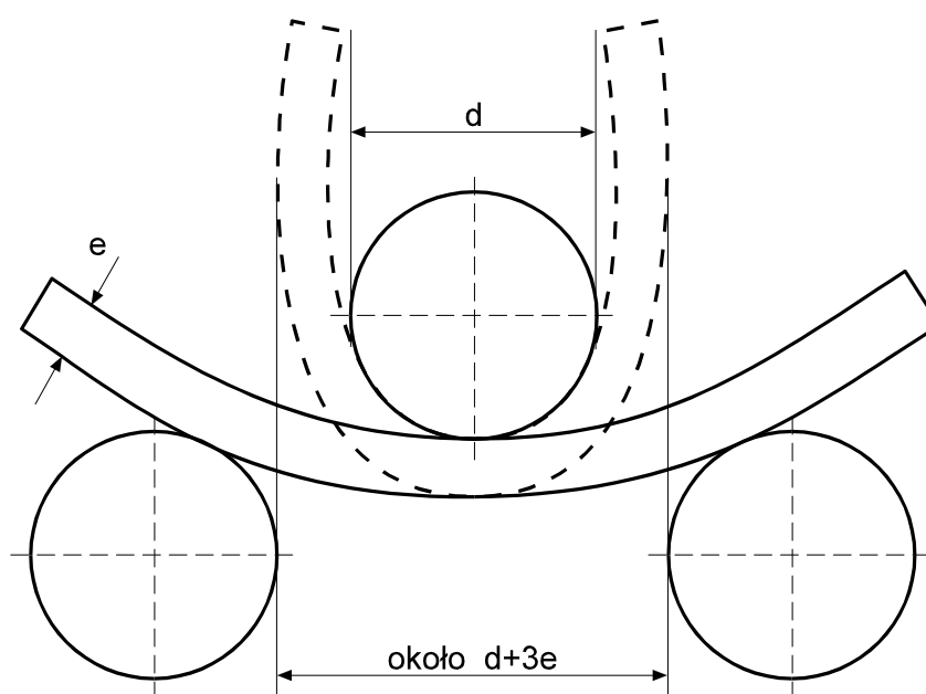
Schemat próby zginania
