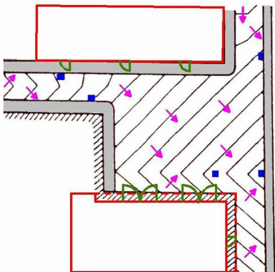
Rys. 4.3.11. Przykłady rozwiązań planów warstwicowych placów
