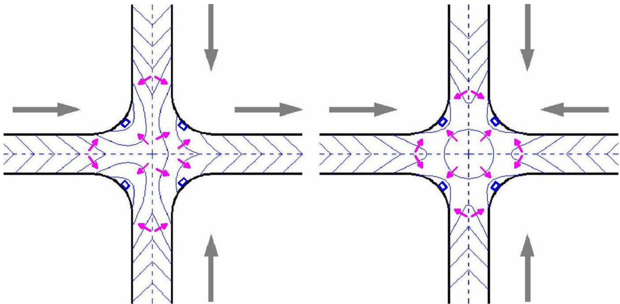
Rys. 4.3.4. Schematy planów warstwowych rozwiązań z tarczą skrzyżowania zlokalizowaną w najniższym punkcie
