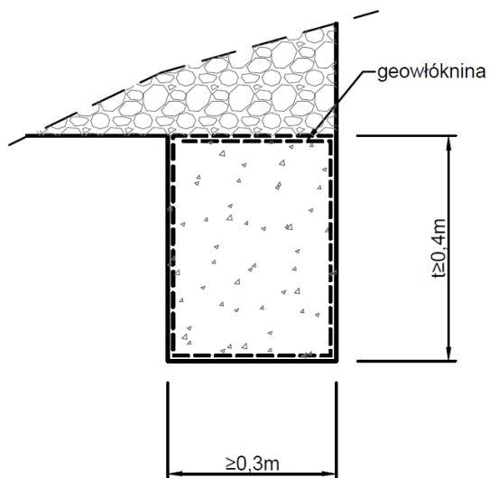
b) dren bez rury drenarskiej z warstwą separacyjną z geosyntetyku (dren francuski)
