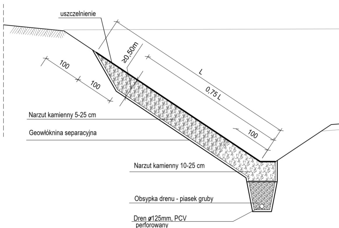
Rys. 5.4.2.1. Przykład ułożenia warstwy odsączającej na skarpi i odprowadzenia wody
