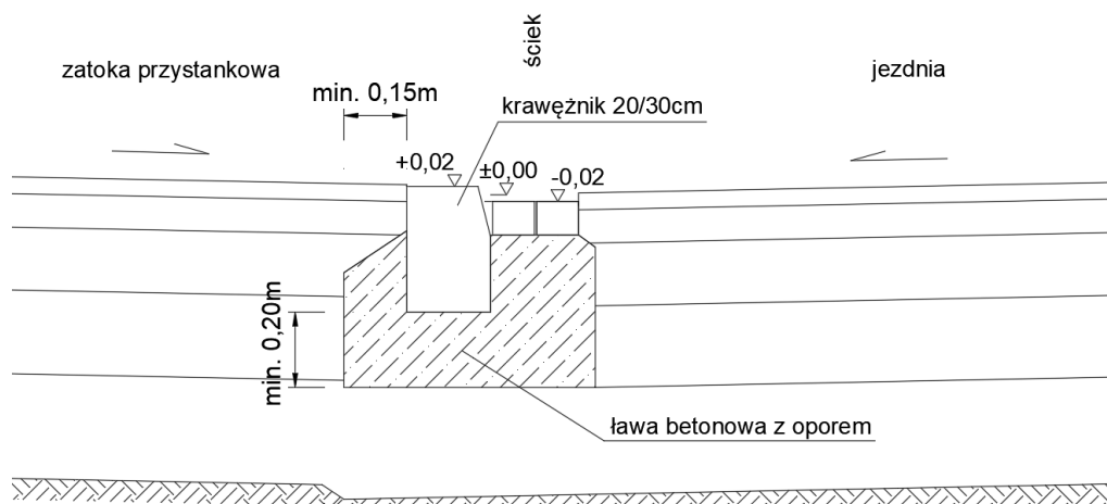
Rys. 4.5.3. Przykłady konstrukcji ścieku na długości zatoki przystankowej
