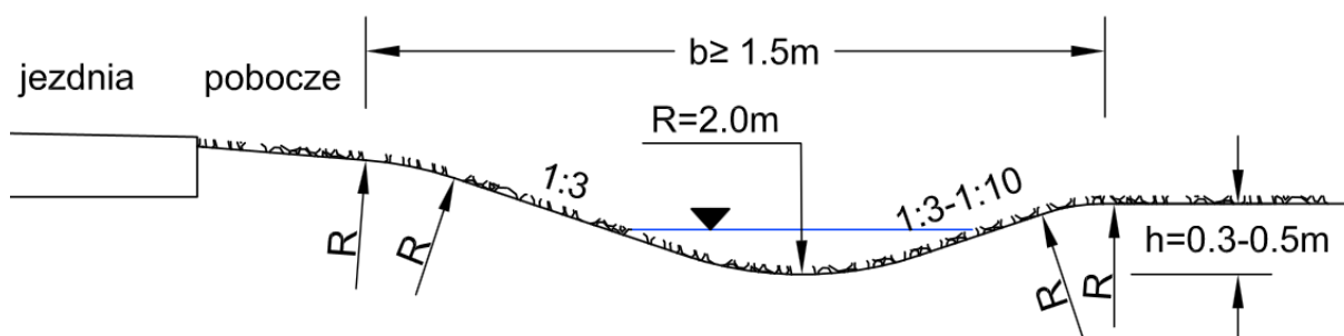
Rys. 4.6.2.6. Przekrój poprzeczny typowego rowu optywowego
