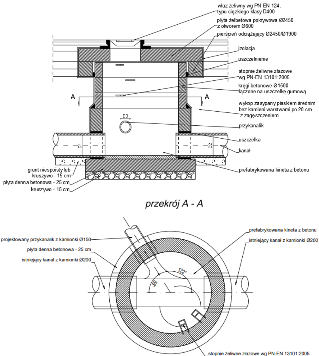
Rys. 4.7.8.2. Przykład studni połączeniowej o głębokości do 3,0 m, umieszczonej w jezdni
