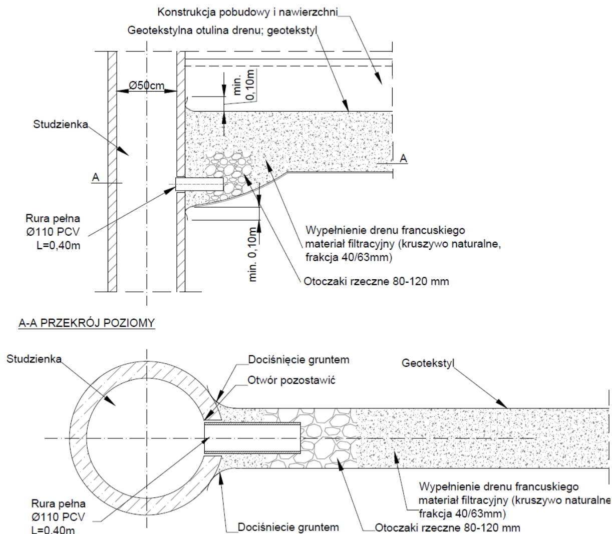
Rys. 5.2.2. Przykład połączenia drenu francuskiego z odbiornikiem (źródło: strona www producenta geosytytyku)
