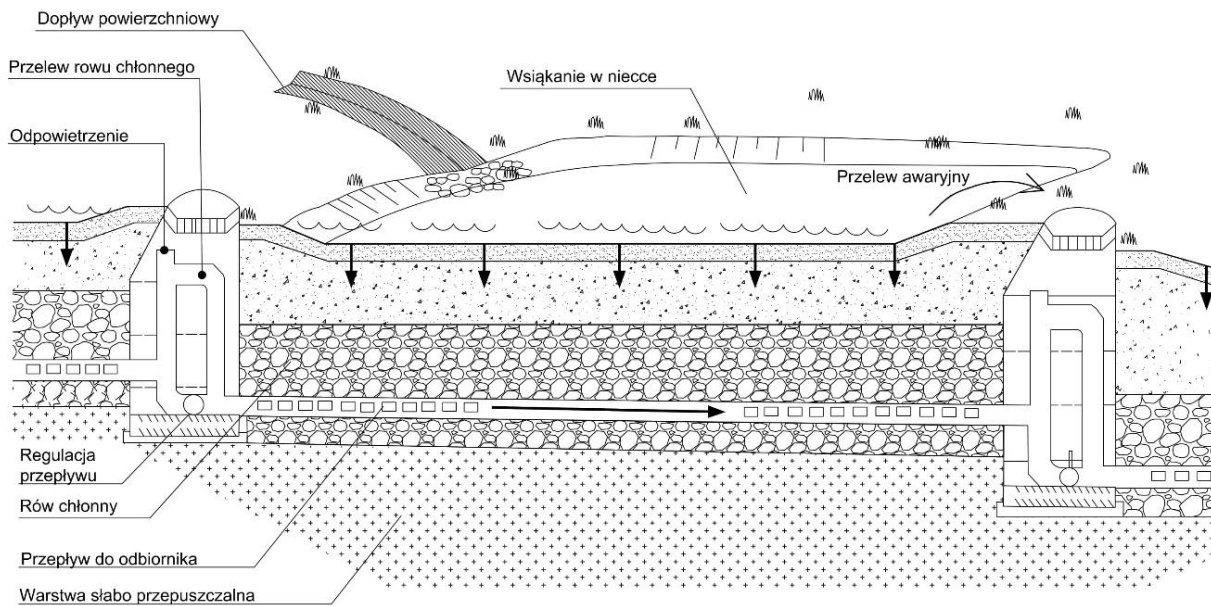
Rys. 8.3.5.1. Przykładowy schemat rozwiązania mieszanego łączącego elementy zbiornika retencyjno-infiltracyjnego oraz filtra pionowego [27]
