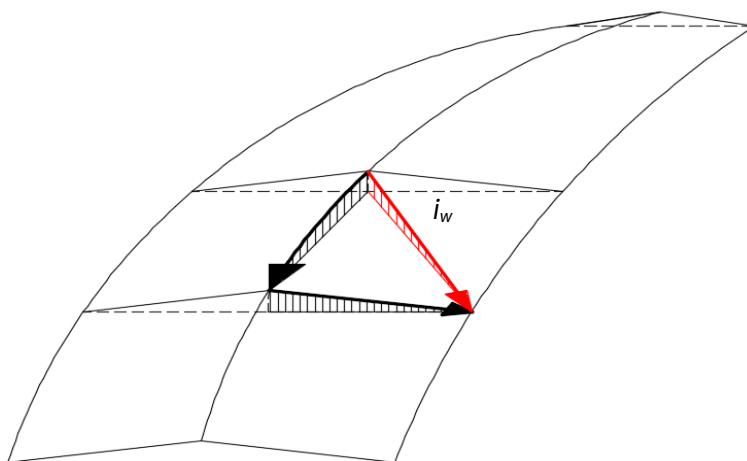
Rys. 4.2.1.2. Ilustracja sptywu wody z jezdni zgodnie ze spadkiem wypadkowym (ukośnym) i_w
