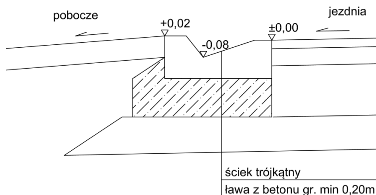
Rys. 4.6.4.10. Przykłady ścieków drogowych i ich zastosowania (1 z 2)
