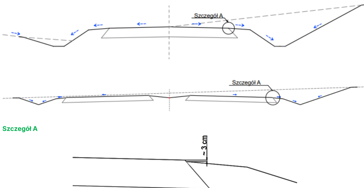
Rys. 4.2.1.1. Schematy odprowadzania wód powierzchniowych i roztopowych w przekroju poprzecznym drogi zamieszkiej
