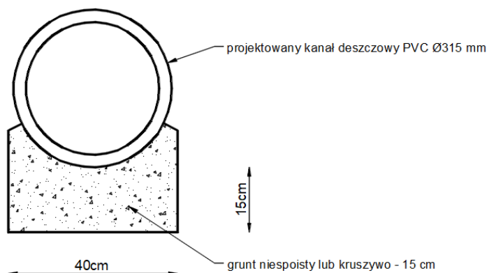
Rys. 4.7.8.1. Przykład posadowienia kanału deszczowego w dobrych warunkach gruntowych
