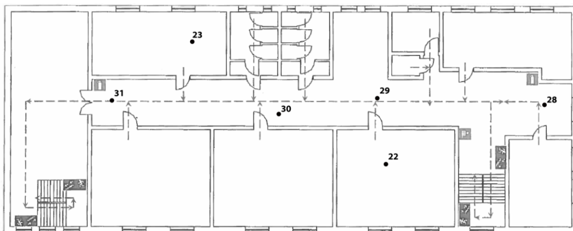
Rys. 1e: Plan rozmieszczenia punktów pomiarowych – 1 piętro, część B
