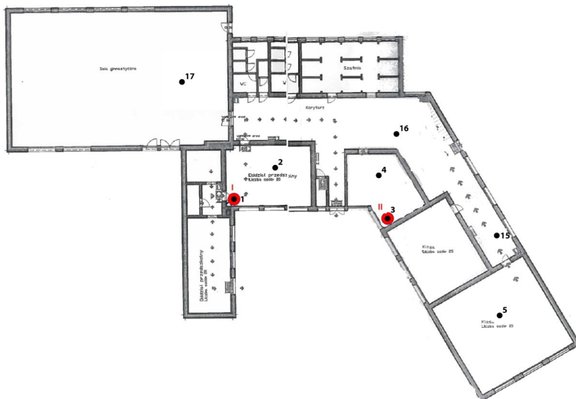
Rys. 1a: Plan rozmieszczenia punktów pomiarowych – parter, część A, kolorem czerwonym oznaczono lokalizację punktów dostępowych
