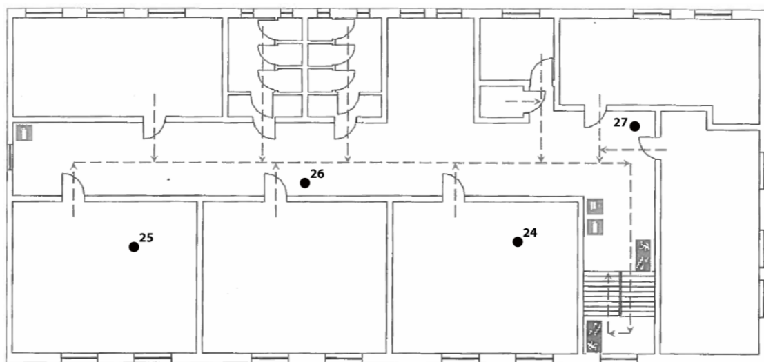
Rys. 1f: Plan rozmieszczenia punktów pomiarowych – 2 piętro, część B
