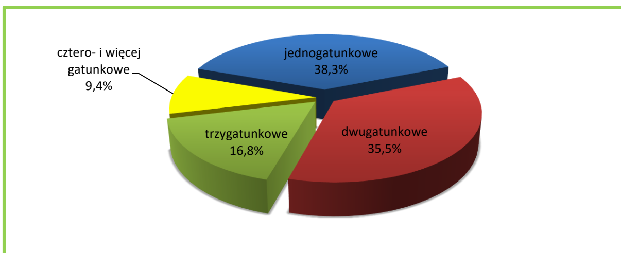
Wykres 4. Charakterystyka bogactwa gatunkowego w Nadleśnictwie
